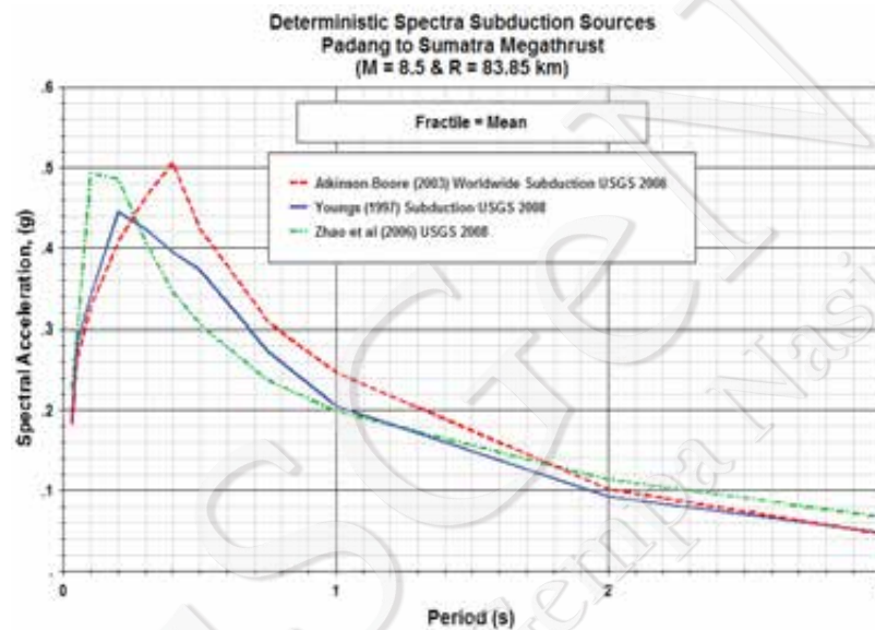
Gambar IV.11. Grafik Respon Spektra untuk sumber gempa Subduksi ( interface )
