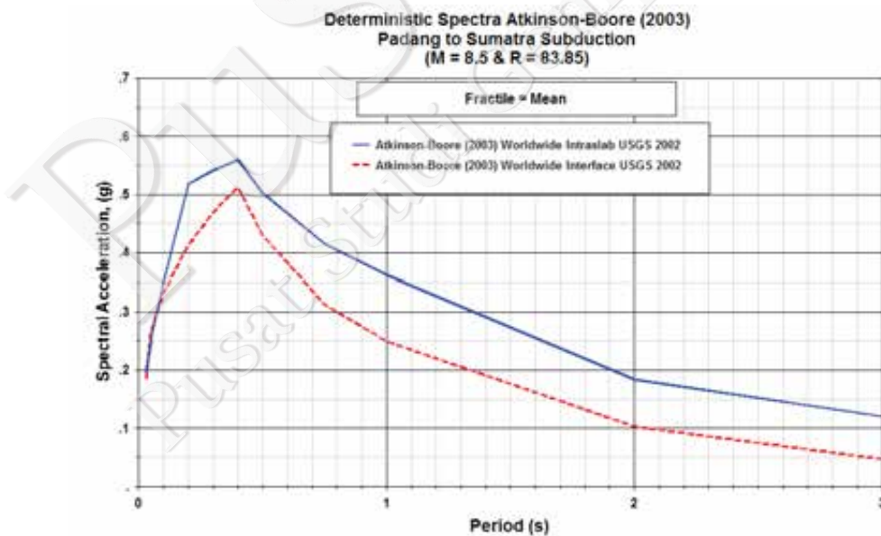
Gambar V-12. Grafik Respon Spektra persamaan GMPE Atkinson-Boore (2003) untuk sumber gempa Deep Background (intraslab) dan Subduksi ( interface ) (Asrurifak, 2010)
