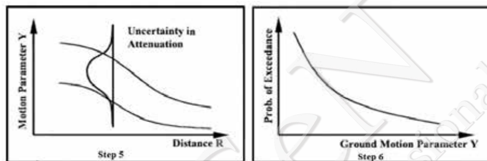
Gambar VI-4. Tahap 5 dan 6 proses Analisis Gempa Probabilistik (PSHA) untuk Peak Ground Acceleration (PGA): Bentuk Kurva Seismic Hazard dan Aplikasinya pada Perkiraan Desain PGA_d untuk Periode Waktu T_d dan Probabilitas Kejadian P_d (Reiter, 1990)
