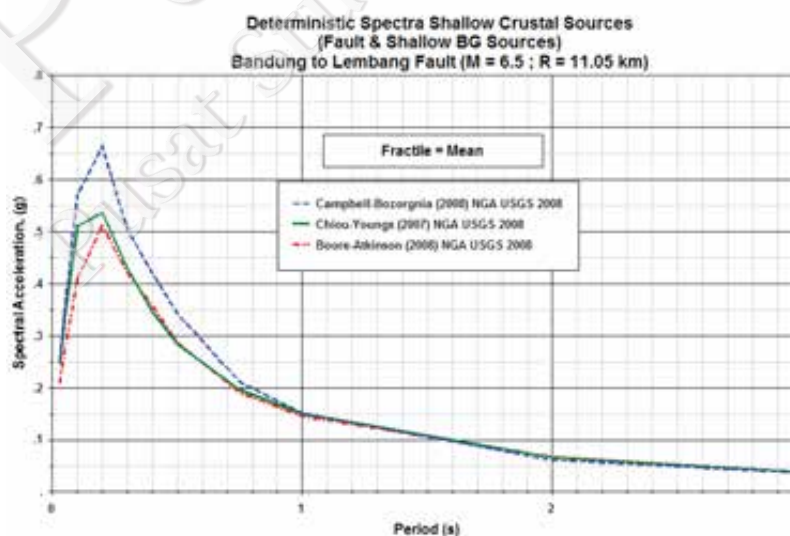
Gambar IV.12. Grafik Respon Spektra untuk sumber gempa Shallow Crustal ( Fault dan Shallow Background ).
