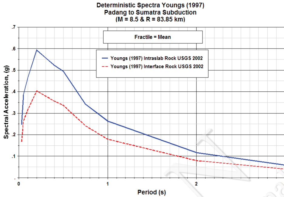
Gambar V-11. Grafik Respon Spektra persamaan GMPE Youngs dkk. (1997) untuk Subduksi Interface dan Benioff Intraslab (Asrurifak, 2010)
