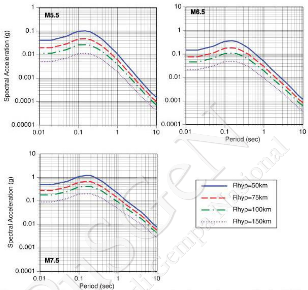
Gambar V-24. Contoh Hasil Perhitungan Median Spektra Percepatan dengan Menggunakan Persamaan GMPE BCHYDRO-2012 untuk Sumber Gempa Subduksi Intraslab dengan Magnitude antara M_w = 5,5 - 7,5 , jarak R_{hypo} antara 50 sampai 150 Km dan nilai V_{s30} = 760 m/s (Abrahamson dkk., 2016)
