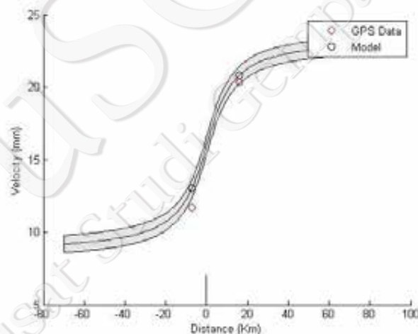
Gambar IV-44. Perhitungan laju geser Sesar Palu-Koro dengan menggunakan metode Simple Screw Dislocation (Savage and Burford, 1973)
