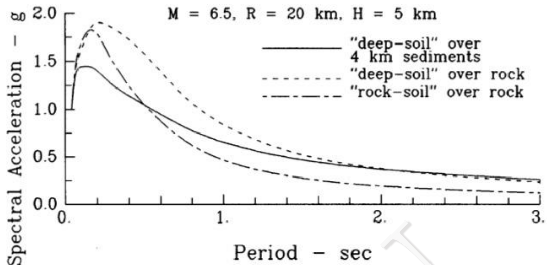
Gambar V-7. Ilustrasi pengaruh jenis tanah terhadap spektral akselerasi suatu gempa (dimodifikasi dari Gupta, 2002)
