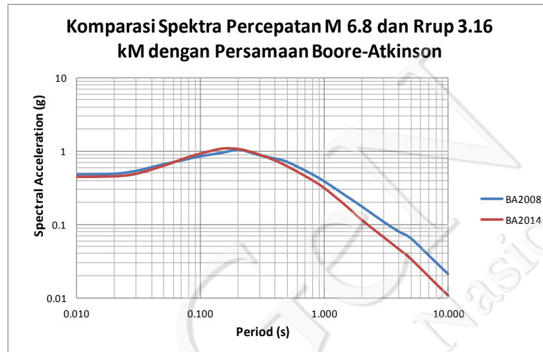
Gambar V-17. Komparasi Nilai Spektra Percepatan Hasil Analisis dengan Menggunakan Persamaan GMPE Boore-Atkinson 2008 dan 2014 (Campbell and Bozorgnia, 2013)
