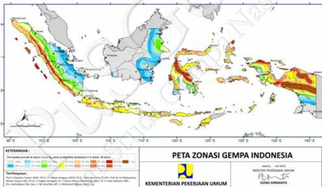
Gambar I-6. Peta Percepatan Puncak di Batuan Dasar Indonesia 2010 untuk Probability of Exceedance 2% dalam 50 tahun (Tim Revisi Peta Gempa Indonesia, 2010)
