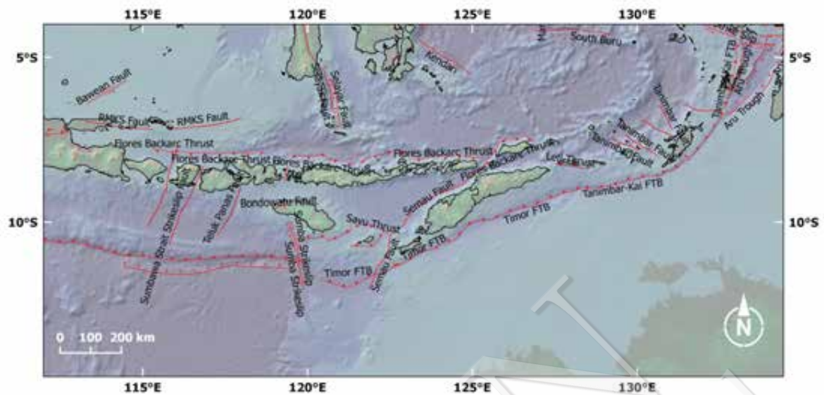
Gambar II-28. Sesar Aktif Daerah Bali-Nusa Tenggara-Banda yang Terangkum Dalam Peta Gempa Nasional 2017
