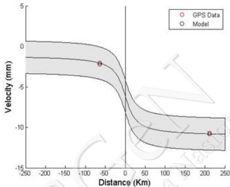
Gambar IV-24. Segmen Dikit-Ketaun
