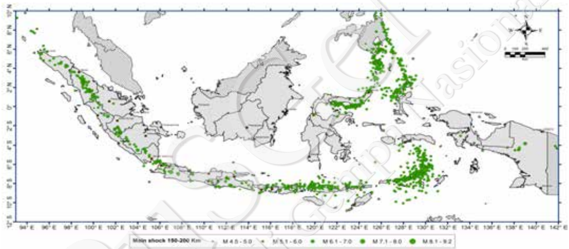
Gambar VI-9. Peta episenter gempa pada kedalaman 150-200 km pada periode 1900-2016 yang digunakan sebagai sumber gempa deep-3 background
