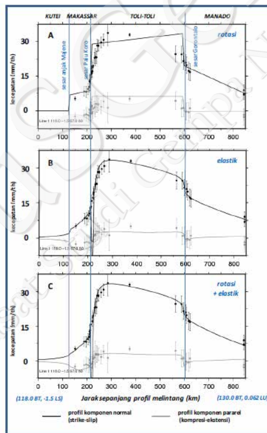
Gambar IV-43. Penampang kecepatan melalui Sesar anjak Majene, Sesar Palu Koro, dan Sesar Gorontalo. Gambar pada bagian atas merupakan penampang kecepatan yang hanya didasarkan pada rotasi rigid-body. Gambar pada bagian tengah merupakan kecepatan yang didasarkan pada model elastik, sedangkan gambar pada bagian bawah merupakan penampang kecepatan yang didasarkan pada kombinasi model rotasi di tengah blok dan elastik di pinggir blok
