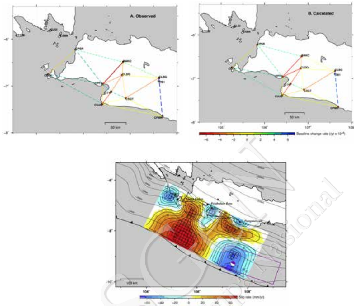
Gambar IV-57. Interplate Coupling di Selat Sunda – Banten - Jawa Bagian Barat (Hanifa dkk., 2014)
