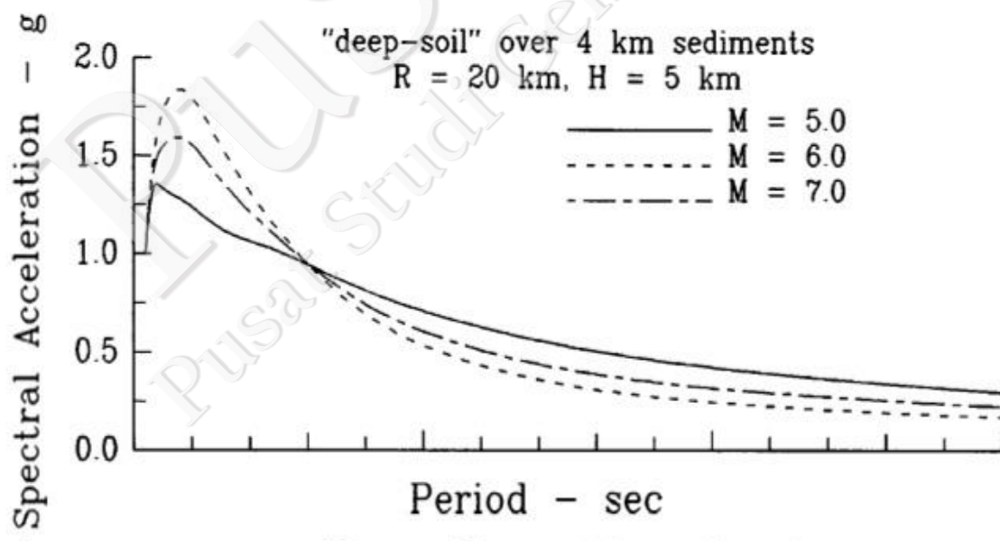
Gambar V-3. Ilustrasi pengaruh magnitude gempa terhadap spectral akselerasi suatu gempa (dimodifikasi dari Gupta, 2002)
