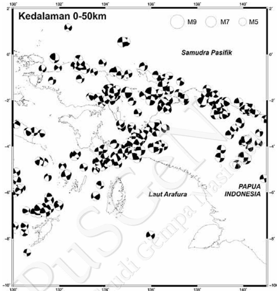
Gambar II-26. Mekanisme fokus gempa dengan magnitudo >5,5 mw memperlihatkan gempa dengan mekanisme sesar mendatar di sekitar Pulau Yapen. Sementara itu, di sekitar Pulau Biak dan pantai utara Kepala Burung didominasi oleh gempa dengan mekanisme sesar naik. Daerah sekitar Manokwari ke selatan sampai dengan Semenanjung Wandamen, gempa yang terjadi beragam dengan mekanisme sesar mendatar dan sesar normal. Data yang digunakan adalah katalog CMT dari tahun 1976 hingga 2013 (Pamumpuni, 2016)
