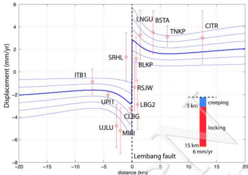
Gambar IV-32 Hasil perhitungan laju geser Sesar Lembang. Titik Merah menunjukkan kecepatan paralel titik GPS terhadap sesar disertai dengan informasi besarnya standar deviasi titik. Kurva berwarna biru merupakan nilai laju geser yang dihitung dengan menggunakan metode Simple Screw Dislocation (Savage and Burford, 1973)
