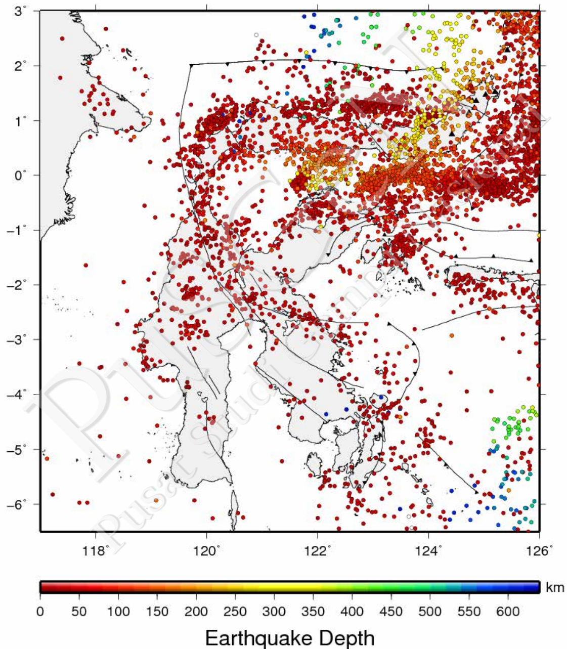
Gambar III-20. Seismisitas dari katalog PuSGeN 2017 di Sulawesi untuk gempa dengan magnitudo \geq 4,5 . Warna menunjukkan kedalaman gempa
