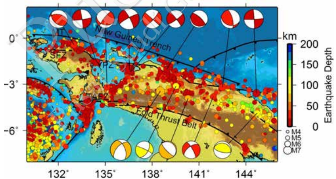
Gambar III-24. Episenter gempa hasil relokasi di zona Papua dan sekitarnya untuk event dengan kedalaman \leq 200 km dan magnitudo \geq 4 . Mekanisme fokus merupakan solusi dari GCMT untuk gempa dengan magnitudo \geq 6 (Shiddiqi, 2015). Singkatan: MT: Manokwari trench , SFZ: zona sesar Sorong, YPZ: zona sesar Yapen, TAFZ: zona sesar Tarera Aiduna. Struktur sesar aktif berdasarkan Sapiie (1998)
