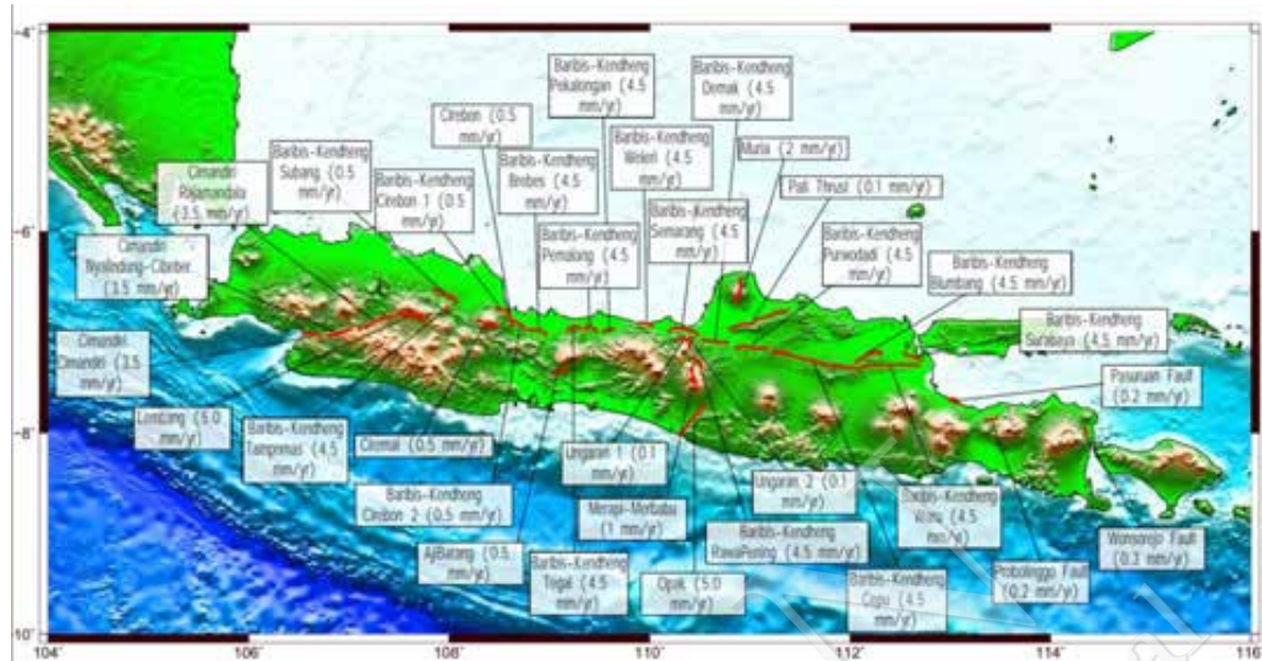
Gambar IV-41. Laju geser segmen-segmen sesar di Jawa
