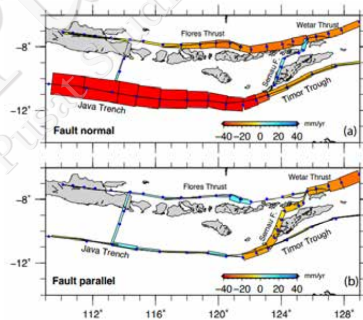
Gambar IV-58. Sliprate Jawa Bagian Timur – NTT (Koulali dkk., 2016a)
