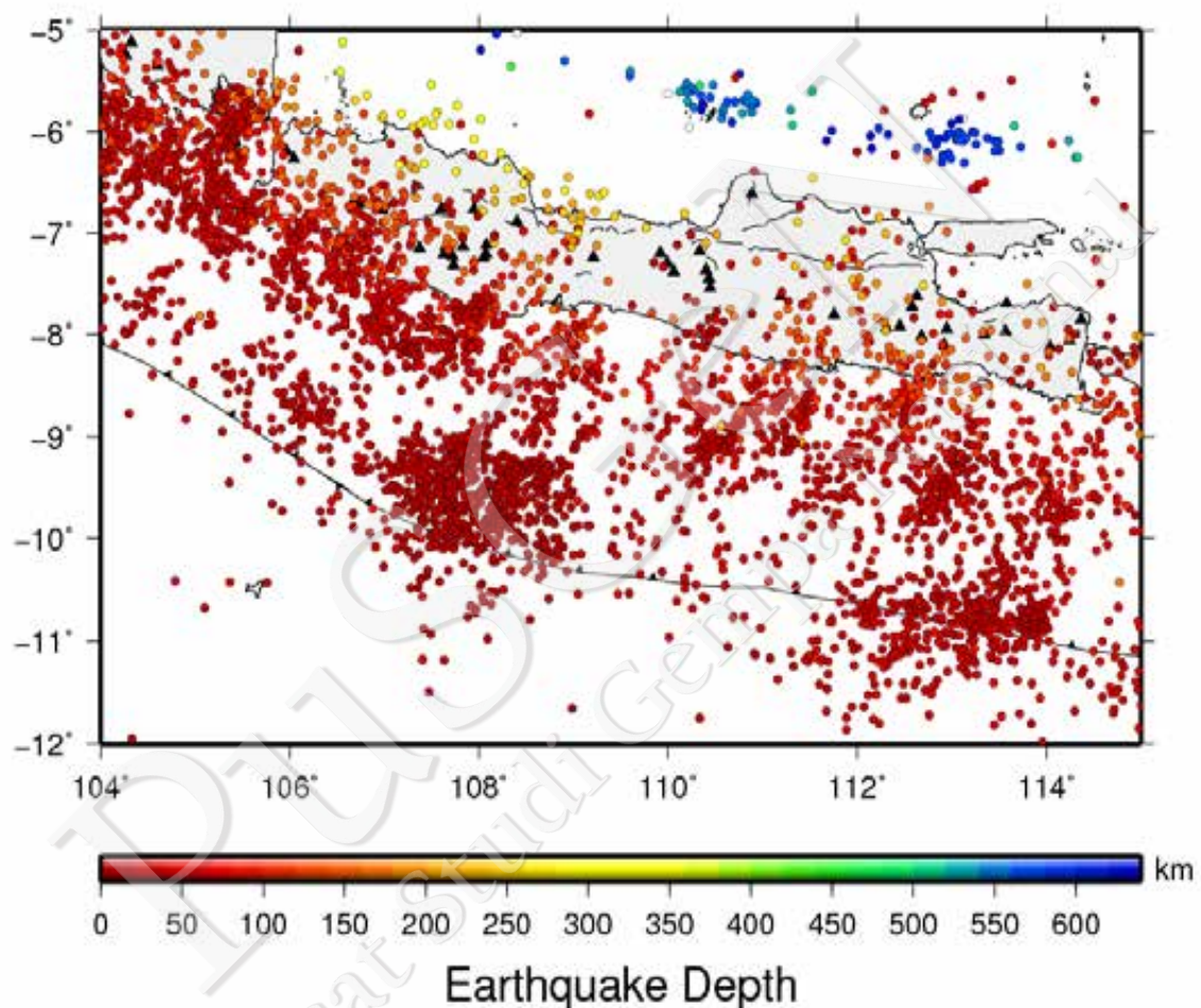
Gambar III-16. Seismisitas dari katalog PuSGeN 2017 di Jawa untuk gempa dengan magnitudo \geq 4,5 . Warna menunjukkan kedalaman gempa
