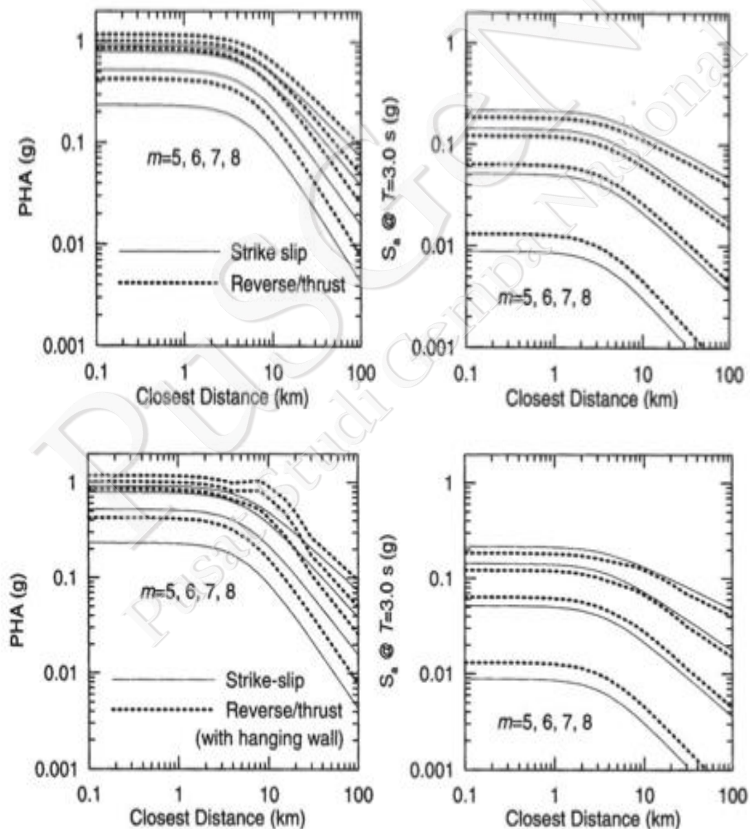
Gambar V-6. Nilai PHA dan spektral akselerasi pada mekanisme sumber gempa ( reverse dan strike-slip ) yang berbeda (Abrahamson dan Silva, 1997)
