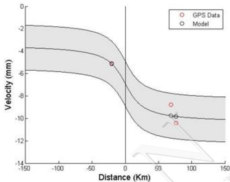
Gambar IV-20. Segmen Renun
