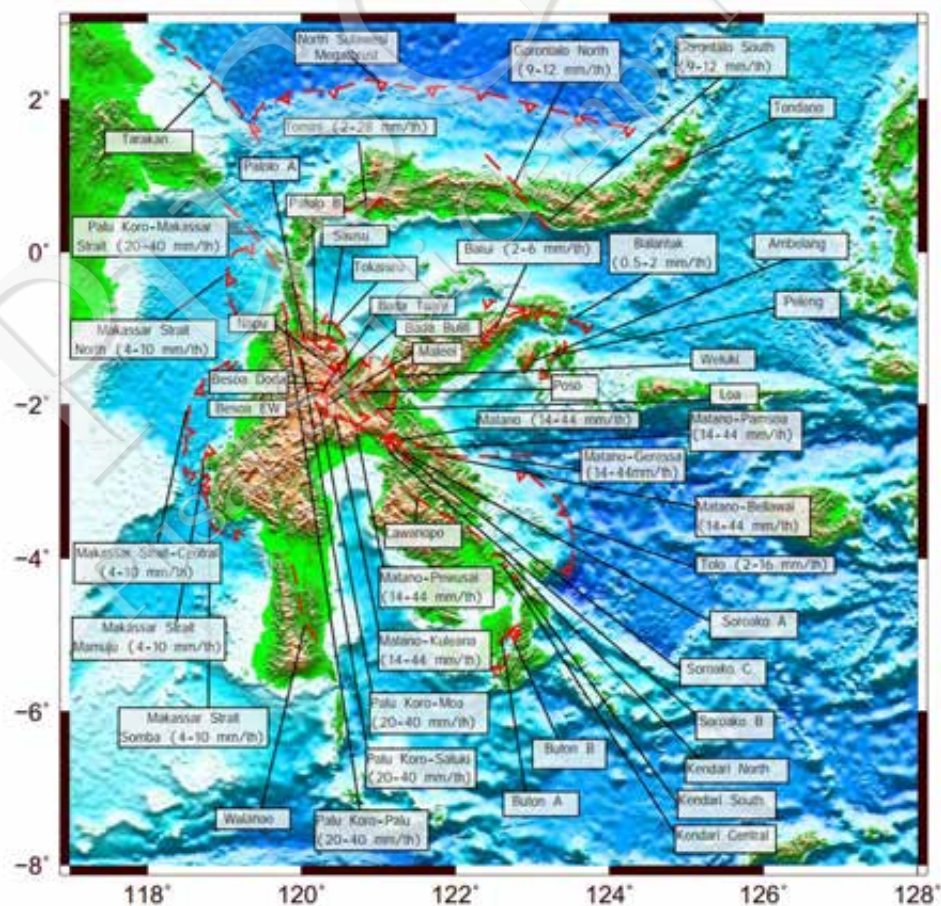
Gambar IV-46. Peta sesar aktif di Sulawesi beserta nilai sliprate -nya
