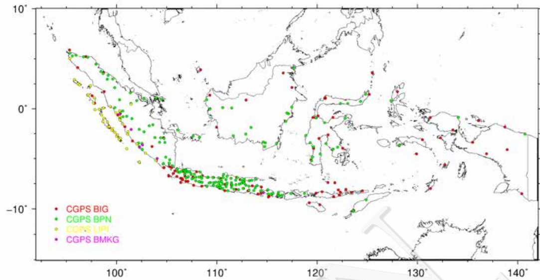
Gambar IV-6. Jaring pengamatan GPS kontinu beberapa instansi di Indonesia
