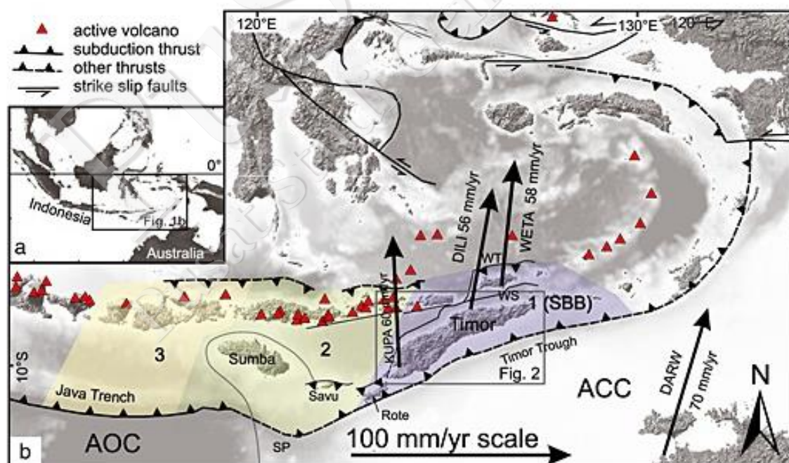
Gambar IV-53. Gambaran umum aktivitas tektonik dan vulkanik di Timor dan Laut Banda (Duffy dkk., 2013)
