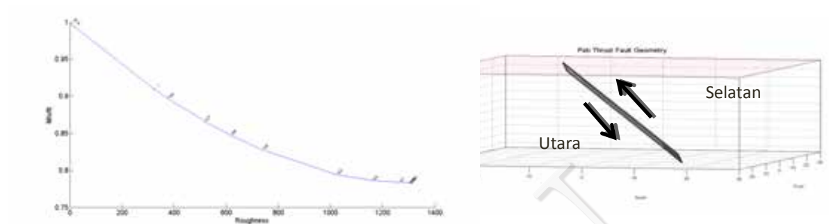
Gambar IV-40. Resolusi model terbaik yang ditunjukkan dengan tanda bintang (kiri) dan model geometri sesar (kanan)
