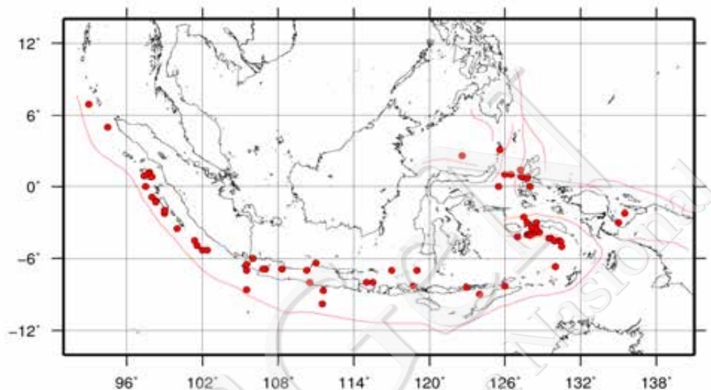
Gambar III-12. Peta episenter gempa M_w \geq 7,0 sebelum tahun 1900 (Musson, 2012)
