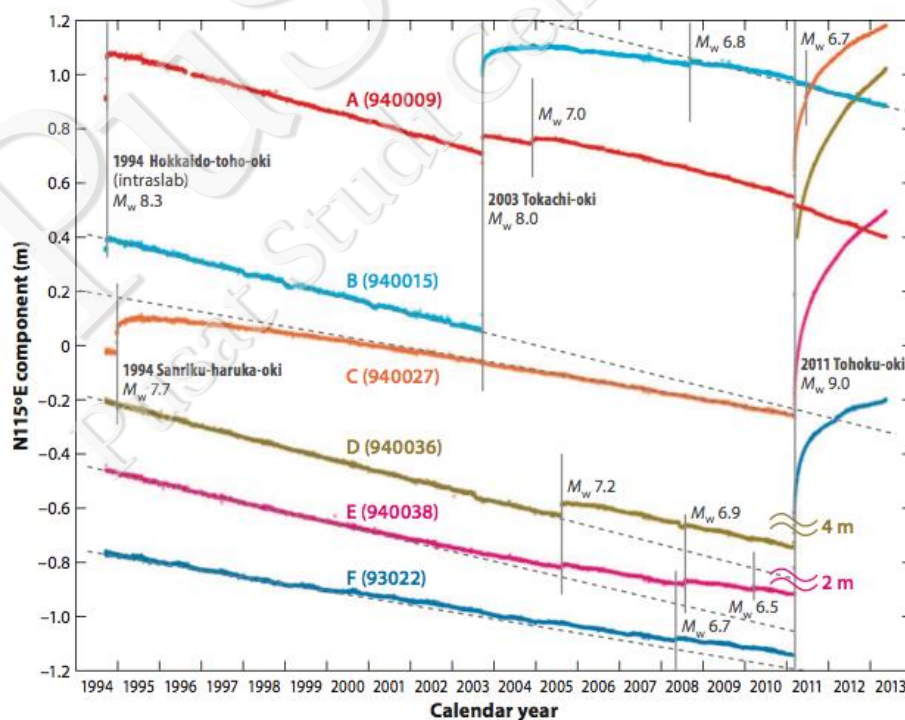
Figure 2.14. Example of time series in GPS data showing the interseismic, coseismic, and postseismic deformation. (Nishimura et al., 2014). Gambar 2.14: Contoh Data time series in GPS data yang menunjukkan pola interseismik (sebelum gempa), coseismik (pada waktu terjadinya gempa), dan postseismik (setelah gempa). (Nishimura et al., 2014). For
