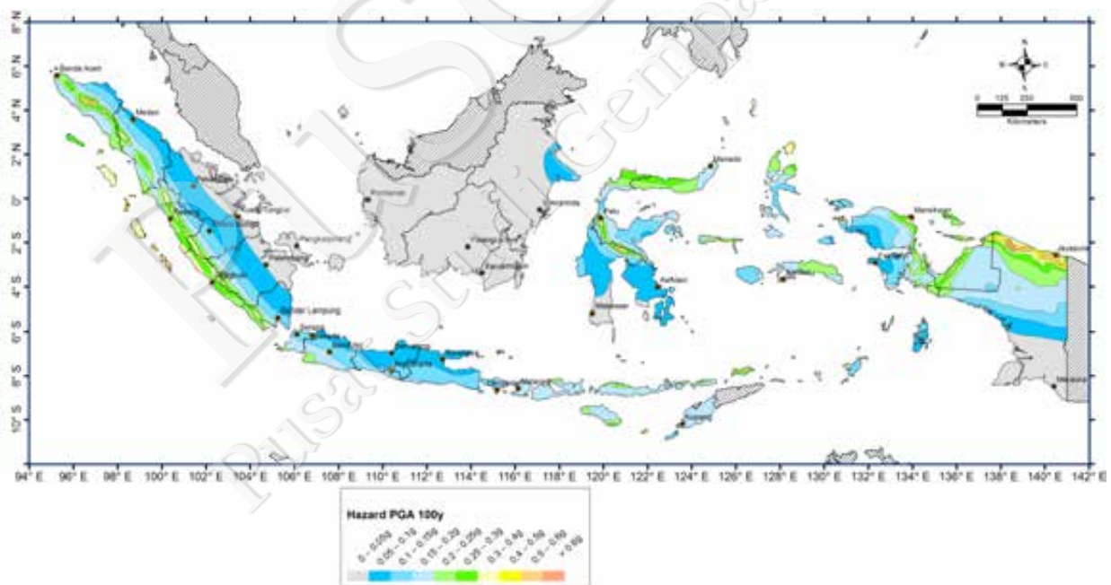
Gambar VI-14. Peta percepatan puncak di batuan dasar (SB) untuk probabilitas terlampaui 10% dalam 10 tahun
