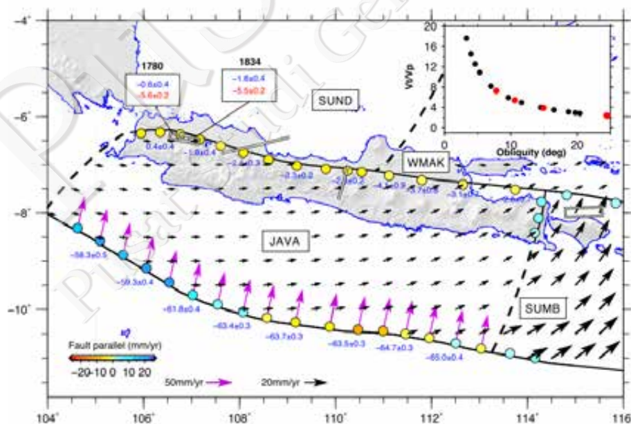
Gambar IV-35. Hasil perhitungan model blok dengan batas Sesar Baribis dan Kendeng. Vektor berwarna hitam merupakan vektor pergerakan model blok sedangkan vektor berwarna magenta yang berada di sepanjang tunjangan palung Jawa merupakan vektor yang tegak lurus terhadap subduksi Jawa. Berdasarkan pemodelan skenario getaran permukaan tanah (Nguyen dkk, 2015) untuk gempa besar ( M_w > 7 ), terdapat segmen Sesar Baribis yang mengalami robekan pada gempa 1780 dan 1834 dengan magnitude gempa sebesar M_w > 7
