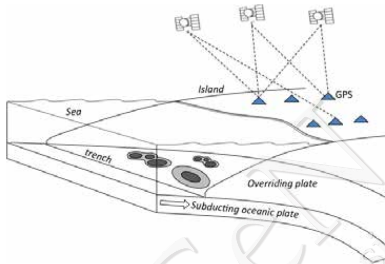
Figure 2.4. Illustration of GPS data to observed crustal deformation in subduction zone. Gambar IV-2: Ilustrasi Pemanfaatan Data GPS untuk Analisis Tektonik. (Hanifa, 2014, yang digambar dengan modifikasi dari Wang dkk., 2012) (re-draw with modification from Wang et al., 2012)
