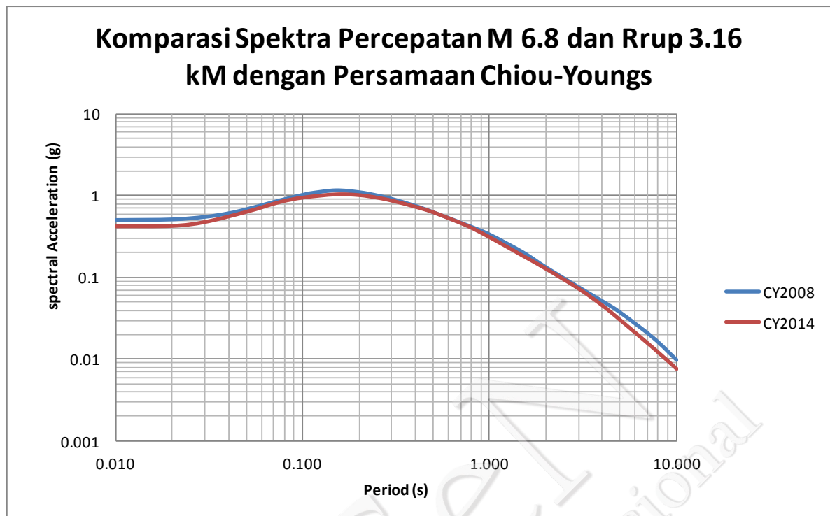
Gambar V-21. Komparasi Nilai Spektra Percepatan Hasil Analisis dengan Menggunakan Persamaan GMPE Chiou-Youngs 2008 dan 2014
