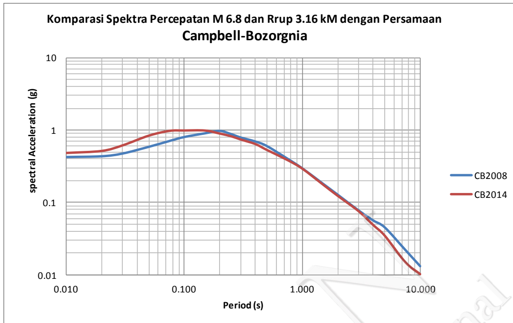
Gambar V-19. Komparasi Nilai Spektra Percepatan Hasil Analisis dengan Menggunakan Persamaan GMPE Campbell-Bozorgnia 2008 dan 2014
