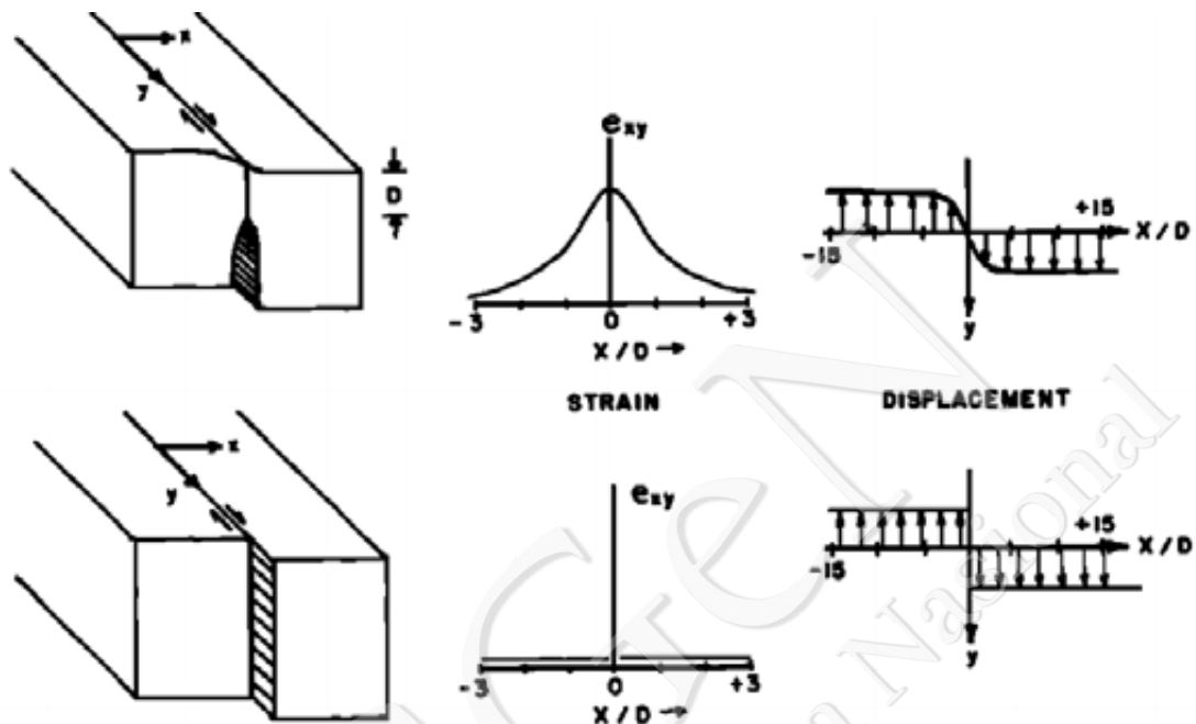
Gambar IV-12. Model sederhana untuk sesar geser yang menunjukkan distribusi regangan geser dan pergeseran horizontal pada permukaan. Gambar pada baris pertama menunjukkan pergeseran permukaan dari sesar geser dengan adanya kuncian pada kedalaman tertentu ( D ) sedangkan gambar pada baris selanjutnya merupakan pergeseran permukaan dari sesar geser dengan asumsi model blok yang memiliki laju geser yang seragam dari permukaan tanah hingga lapisan elastis (Savage dan Burford, 1973)
