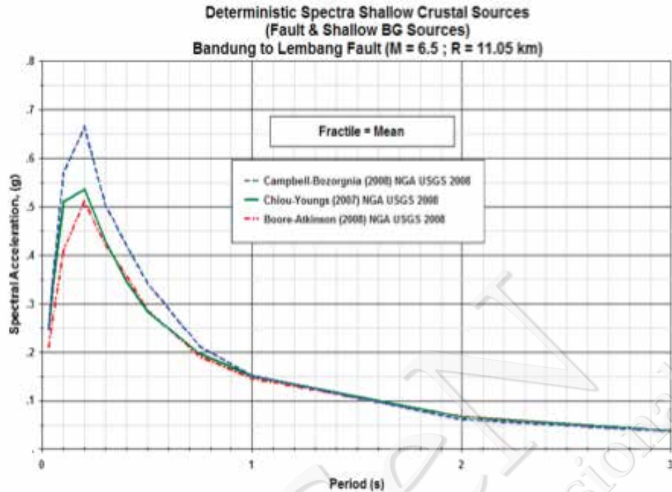
Gambar V-10. Grafik respon spektra atenuasi Boore-Atkinson (2008), Campbell-Bozorgnia (2008) dan Chiou-Youngs (2008) untuk sumber gempa shallow crustal ( shallow background dan fault ) (Asrurifak, 2010)
