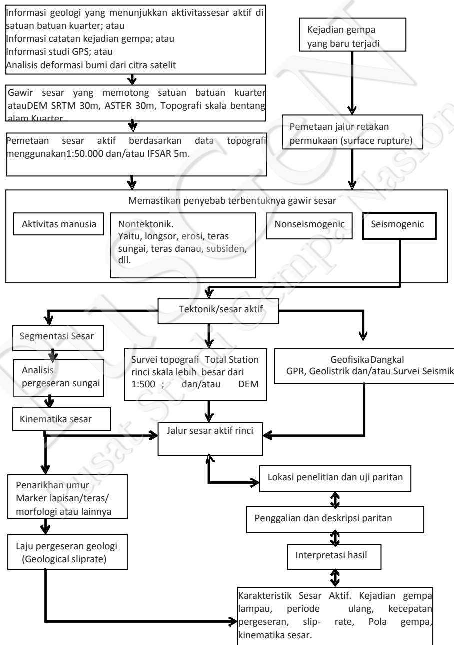
Gambar II-2. Diagram Penelitian Metode Paleoseismologi Di Wilayah Tropis Indonesia (Daryono, 2016; McCalpin, 1996)
