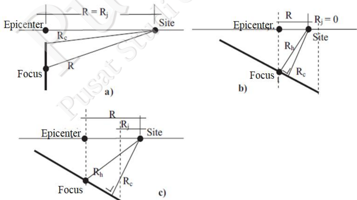
Gambar V-5. Ilustrasi definisi jarak sumber gempa ke lokasi (berdasarkan Asrurifak, 2010): a) jarak proyeksi sesar ke site jauh, b) jarak proyeksi sesar ke site memotong, c) jarak proyeksi sesar ke site dekat
