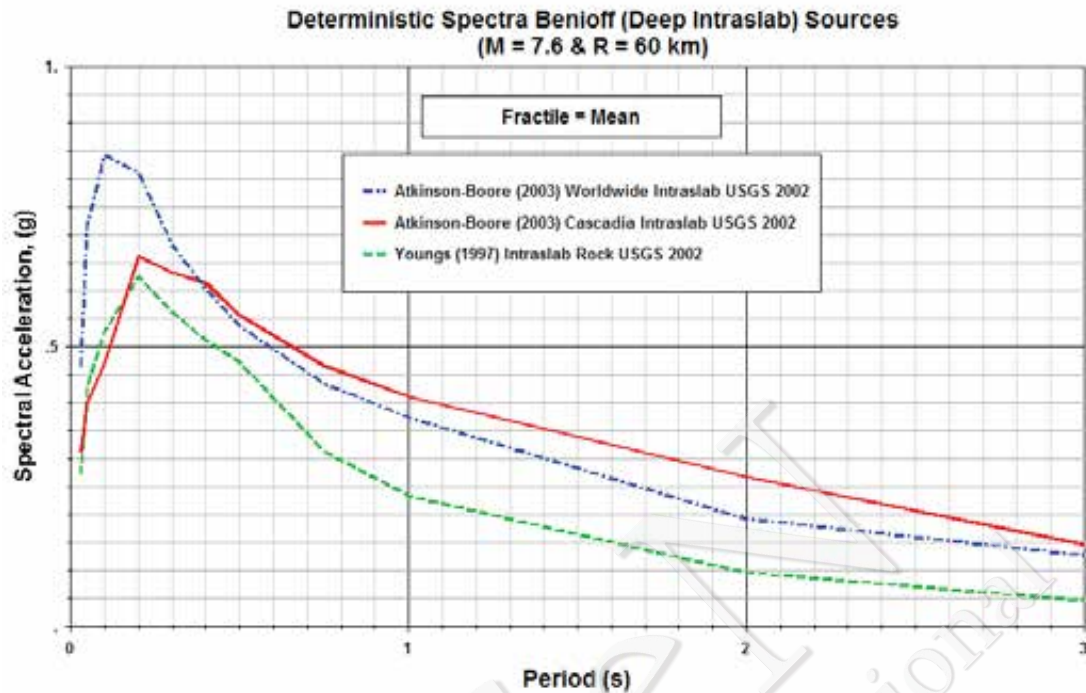
Gambar IV.13. Grafik Respon Spektra untuk sumber gempa Benioff (Deep Background / intralab) (Asrurifak, 2010)
