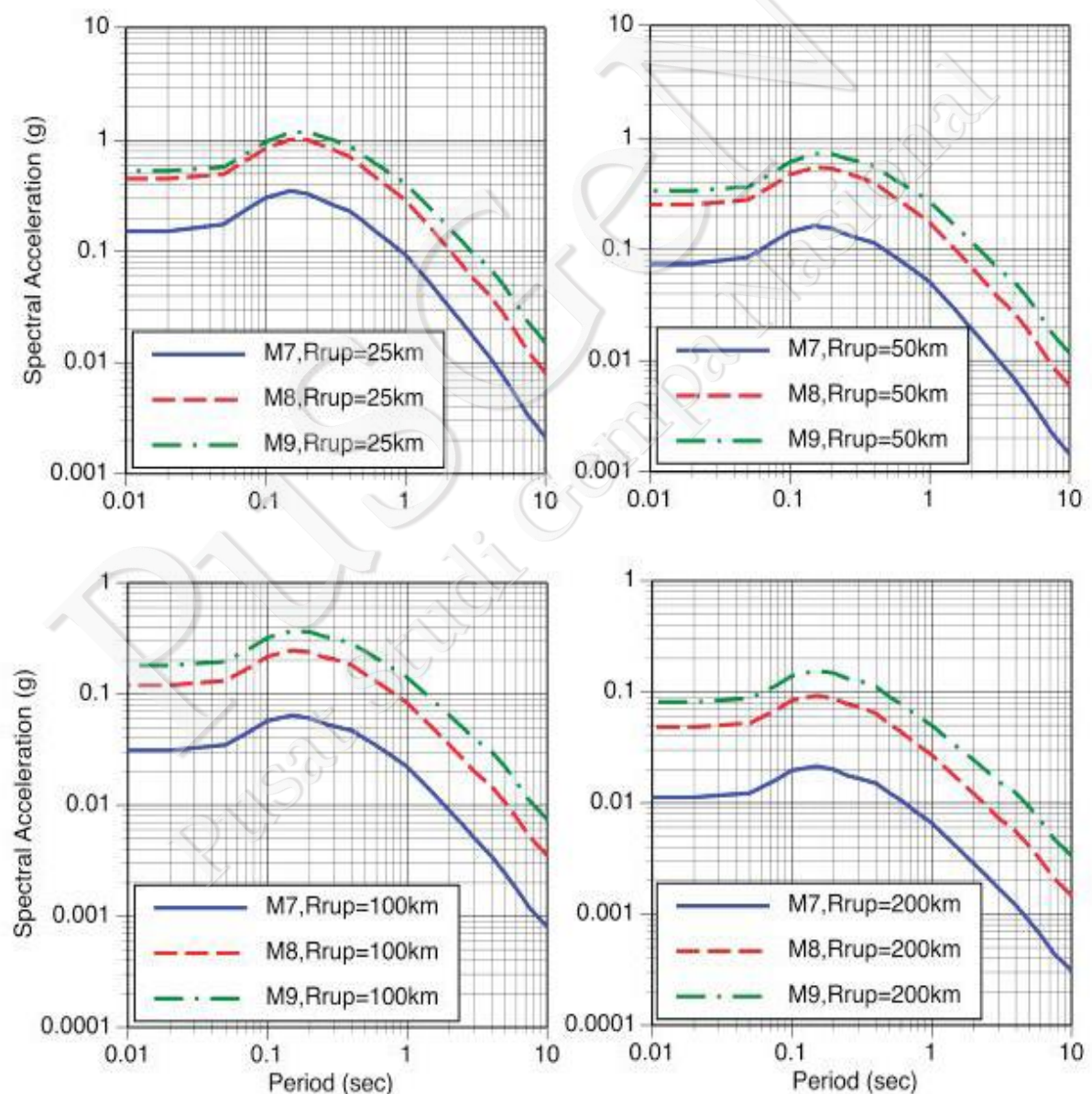
Gambar V-23. Contoh Hasil Perhitungan Median Spektra Percepatan dengan Menggunakan Persamaan GMPE BCHYDRO-2012 untuk Sumber Gempa Subduksi Interface dengan Magnitude antara M_w = 7 - 9 , jarak R_{rup} antara 25-200 Km dan nilai V_{S30} = 760 m/s (Abrahamson dkk., 2016)
