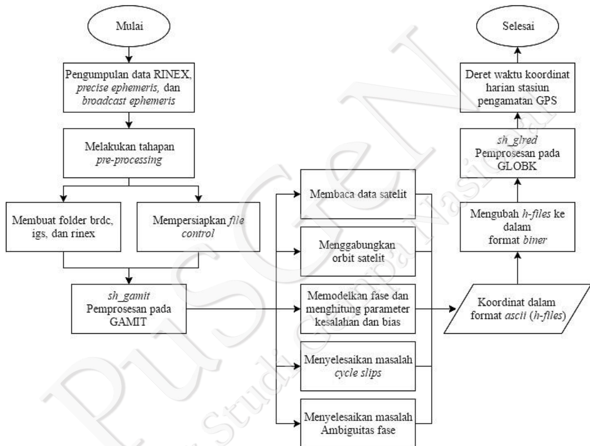
Gambar IV-8. Diagram alir pengolahan dengan software GAMIT/GLOBK
