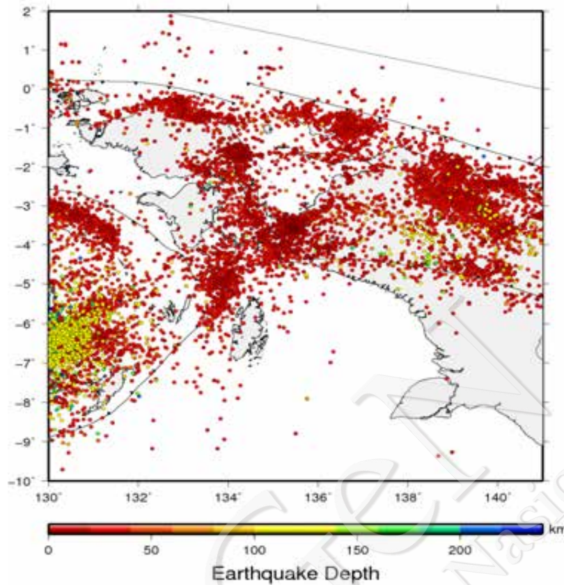
Gambar III-23. Seismisitas dari katalog PuSGeN 2017 di Papua untuk gempa dengan magnitudo \geq 4,5 . Warna menunjukkan kedalaman gempa
