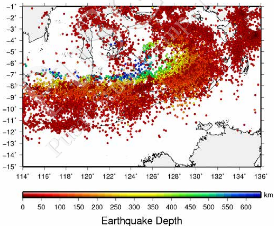
Gambar III-28. Seismisitas dari katalog PuSGeN 2017 di Bali, Nusa Tenggara, dan Laut Banda untuk gempa dengan magnitudo \geq 4,5 . Warna menunjukkan kedalaman gempa
