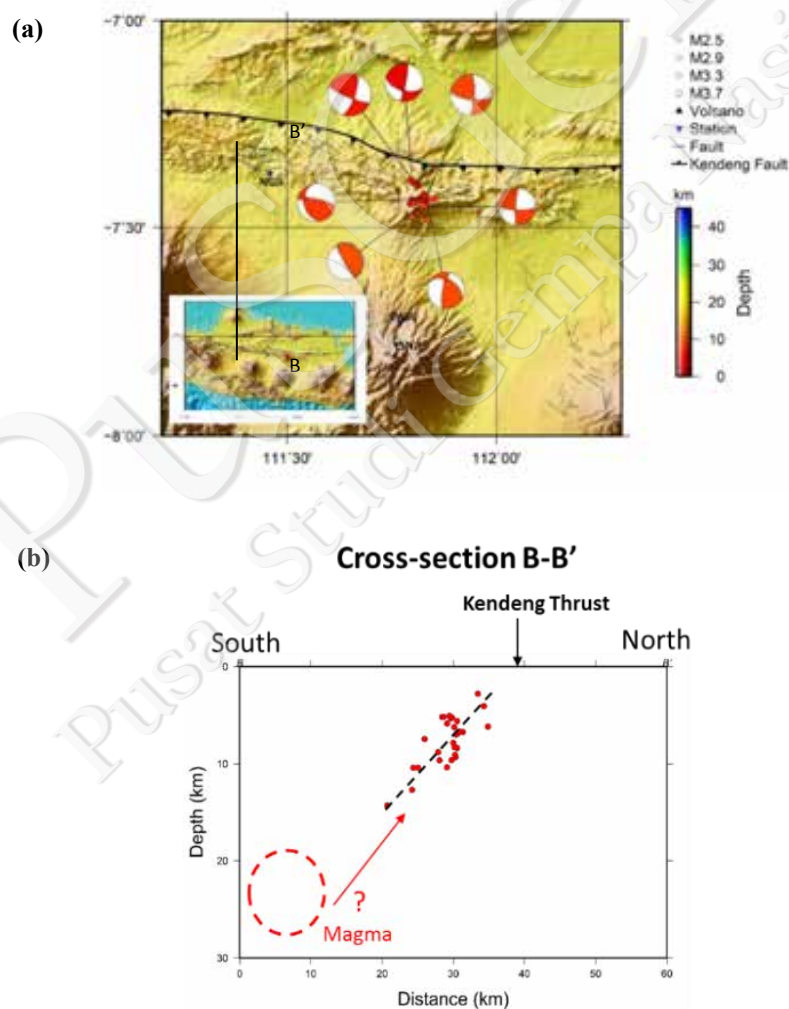
Gambar III-19. a) Peta episenter dan mekanisme fokus gempa hasil relokasi di Madiun selama bulan Februari 2016 dengan kedalaman dangkal \leq 30 km. Lingkaran merah sampai kuning adalah hiposenter gempa berdasarkan kedalaman. Segitiga terbalik warna biru adalah stasiun seismik BMKG yang digunakan b) Penampang vertikal B-B' dari gempa-gempa di Madiun (Nugraha dkk., 2017 in prep. )
