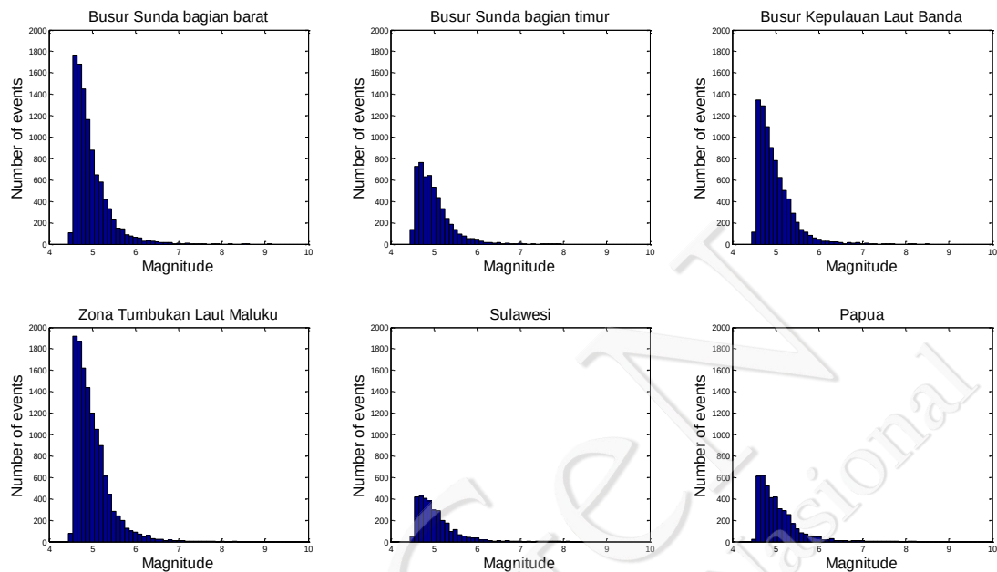
Gambar III-9. Histogram magnitudo gempa untuk beberapa zona tektonik di Indonesia
