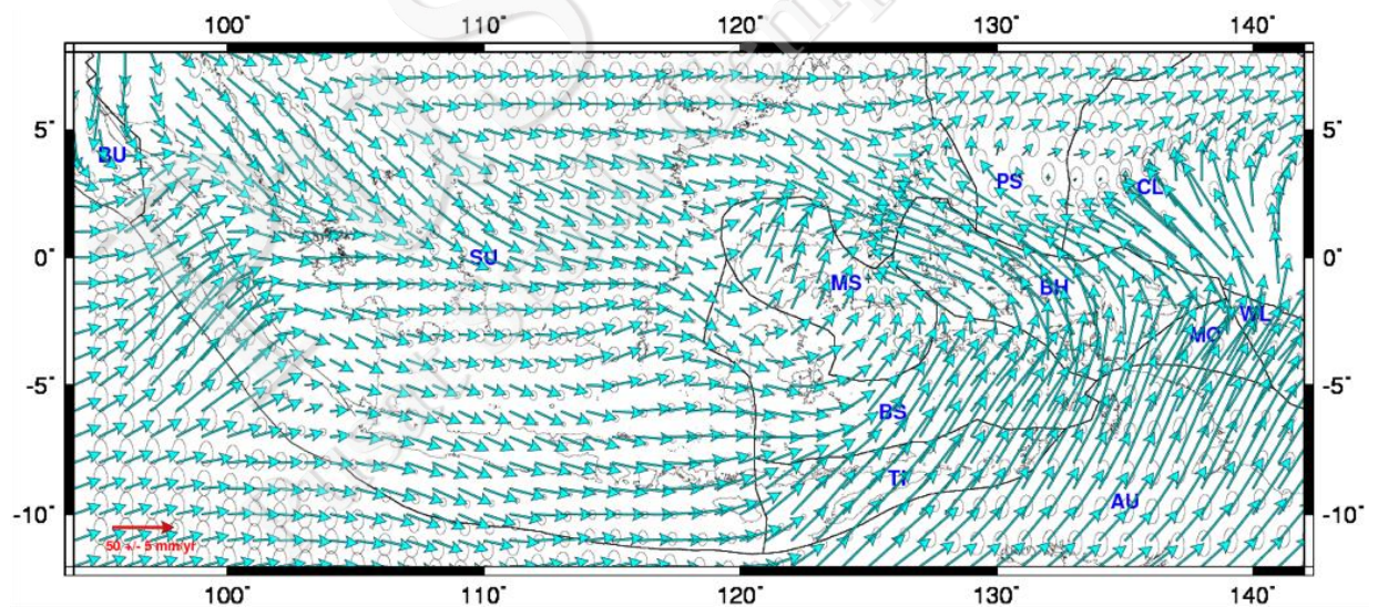
Gambar IV-14. Block Rotation Model di Indonesia dari data GPS (Wibowo, 2016)
