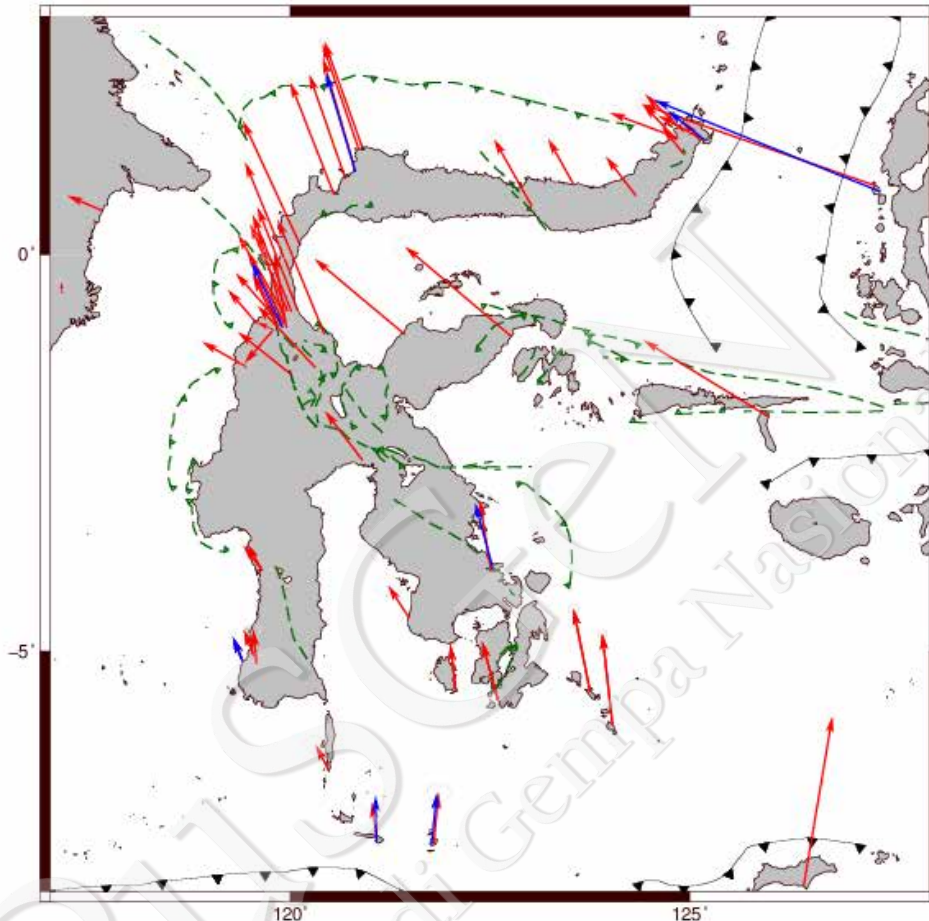
Gambar IV-42. Tektonik Sulawesi dan Peta kecepatan deformasi di Sulawesi dari data GPS (Susilo dkk., 2016)
