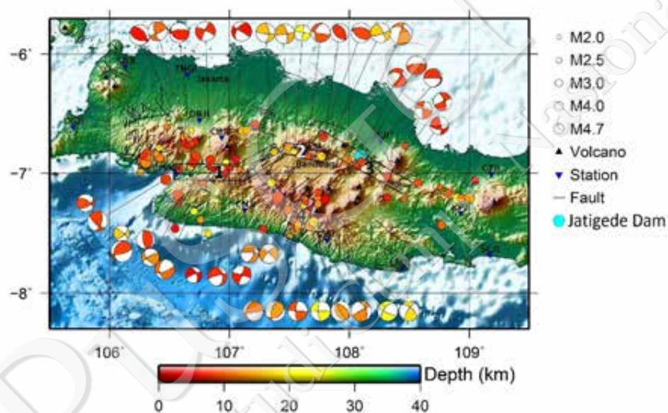
Gambar III-18. Peta episenter dan mekanisme fokus gempa di Jawa Barat. Perbedaan warna menunjukkan kedalaman yang berbeda. Kotak nomor satu sampai empat adalah klaster gempa yang kemungkinan berasosiasi dengan sesar di Jawa Barat (Supendi dkk., 2016)
