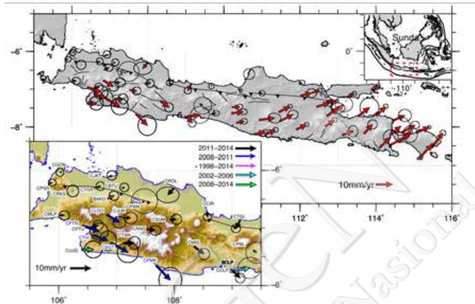
Gambar IV-34. Persebaran titik GPS yang digunakan dalam perhitungan model blok Sesar Baribis dan Kendeng (Koulali dkk, 2016b)
