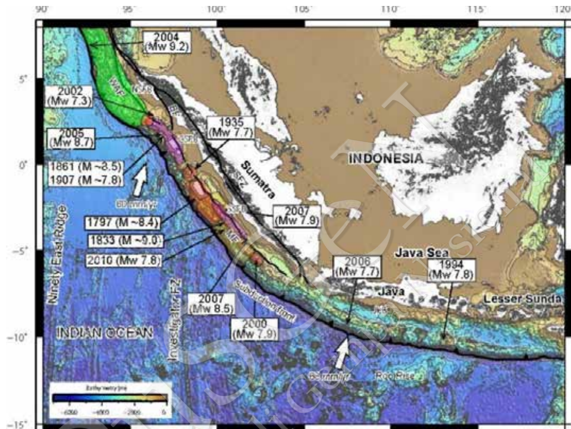
Gambar II-3. Peta regional struktur yang berkembang di Sumatra (Diament dkk., 1992; Malod and Kemal, 1996; Samuel and Harbury, 1996), dan daerah rupture gempa besar (Abercrombie dkk., 2001; Ammon dkk., 2006; Briggs dkk., 2006), serta fitur struktur utama di kerak samudra
