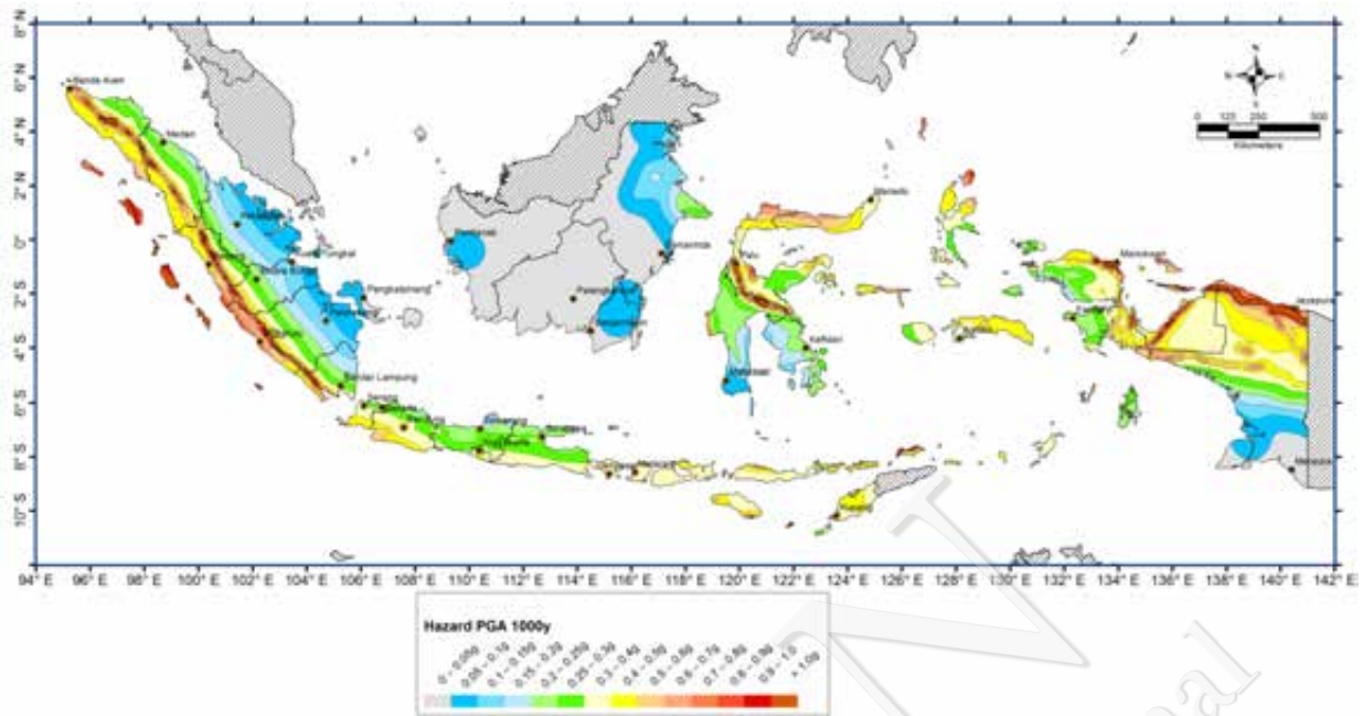
Gambar VI-17. Peta percepatan puncak di batuan dasar (SB) untuk probabilitas terlampaui 7% dalam 75 tahun
