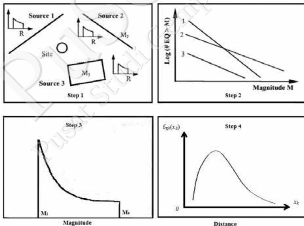
Gambar VI-3. Tahap 1-4 dari Analisis Risiko Gempa Probabilistik (PSHA) untuk Peak Ground Acceleration (PGA) : Bentuk Kurva Seismic Hazard dan Aplikasinya pada Perkiraan Desain PGA_d untuk Periode Waktu T_d dan Probabilitas Kejadian P_d (Digambar ulang dari Reiter, 1990)
