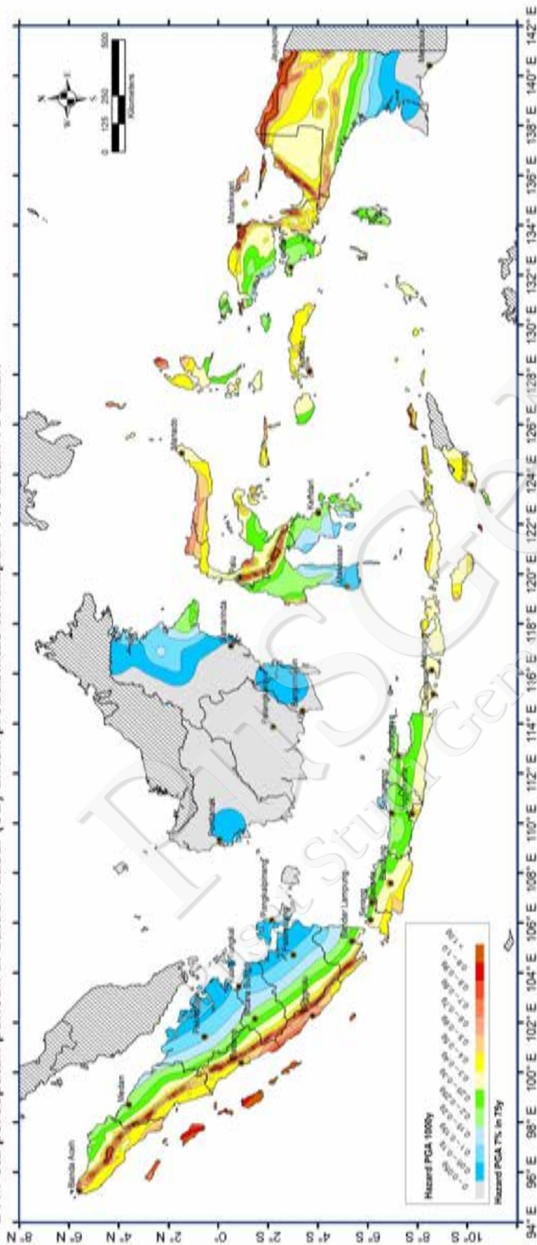
D7: Peta percepatan puncak di batuan dasar (SB) untuk probabilitas terlampaui 7% dalam 75 tahun
