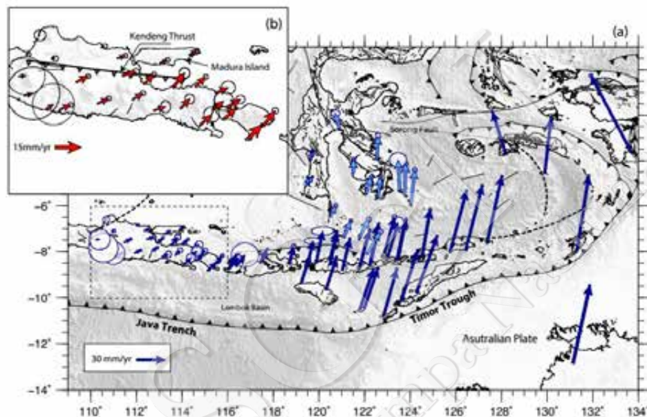
Gambar IV-39. Persebaran titik GPS di sekitar Sesar Kendeng. Garis hitam mengindikasikan letak sesar dan vektor berwarna merah merupakan vektor pengamatan GPS. Tampak bahwa vektor kecepatan titik GPS yang berada di sekitar sesar memiliki nilai yang pola yang semakin mengecil kecepatannya dari selatan ke utara sesar (Koulali dkk, 2016a)
