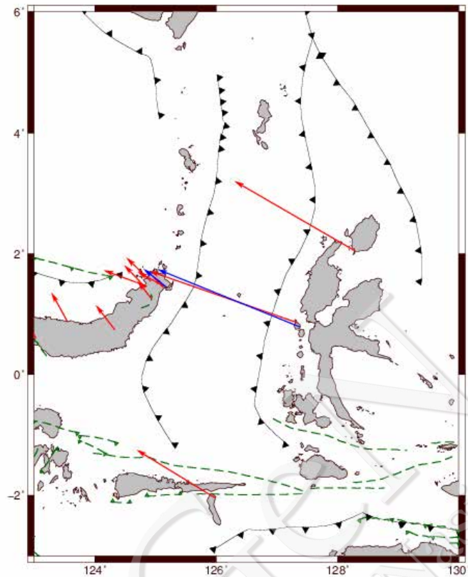
Gambar IV-49. Distribusi titik-titik GPS di Halmahera dan sekitarnya (Susilo dkk. 2016)
