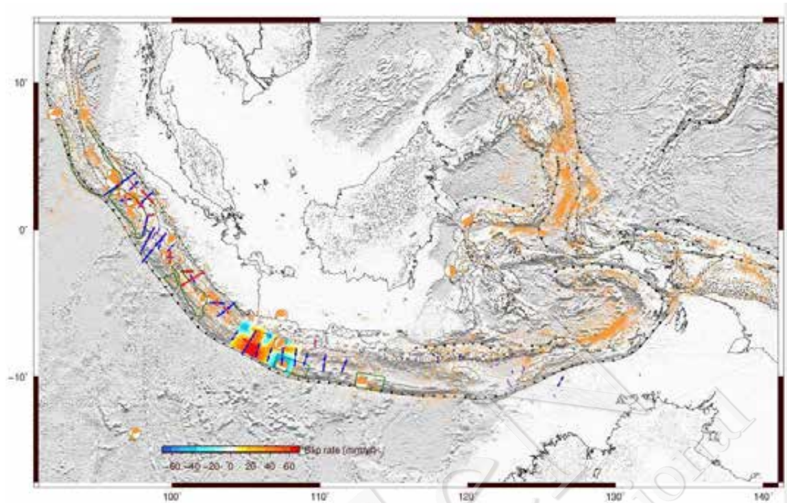
Gambar IV-60. Perhitungan regangan. Warna merah di selatan Jawa Bagian Barat memperlihatkan interplate coupling , warna oranye adalah seismisitas dari katalog PuSGeN 2016
