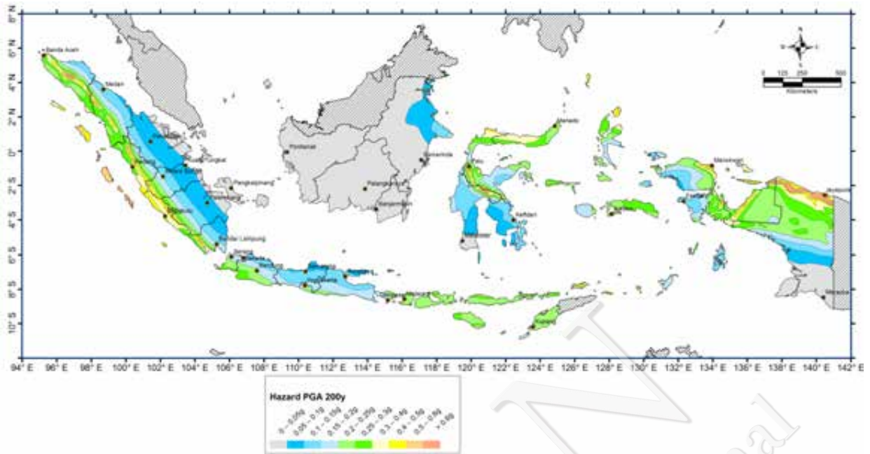
Gambar VI-15. Peta percepatan puncak di batuan dasar (SB) untuk probabilitas terlampaui 5% dalam 10 tahun
