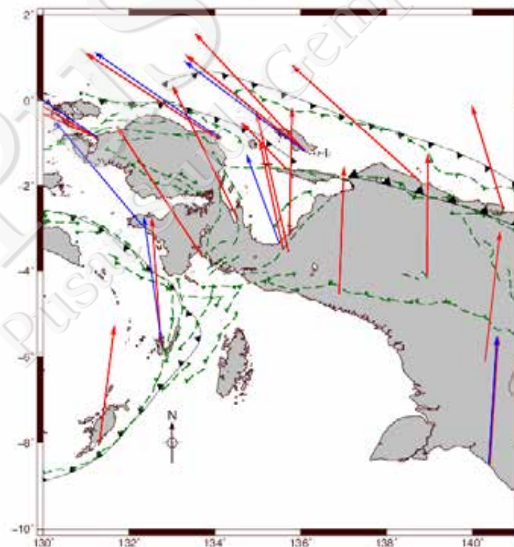
Gambar IV-52. Distribusi stasiun GPS di Papua yang terdiri atas GPS berkala dan GPS kontinyu. (Susilo dkk. 2016)
