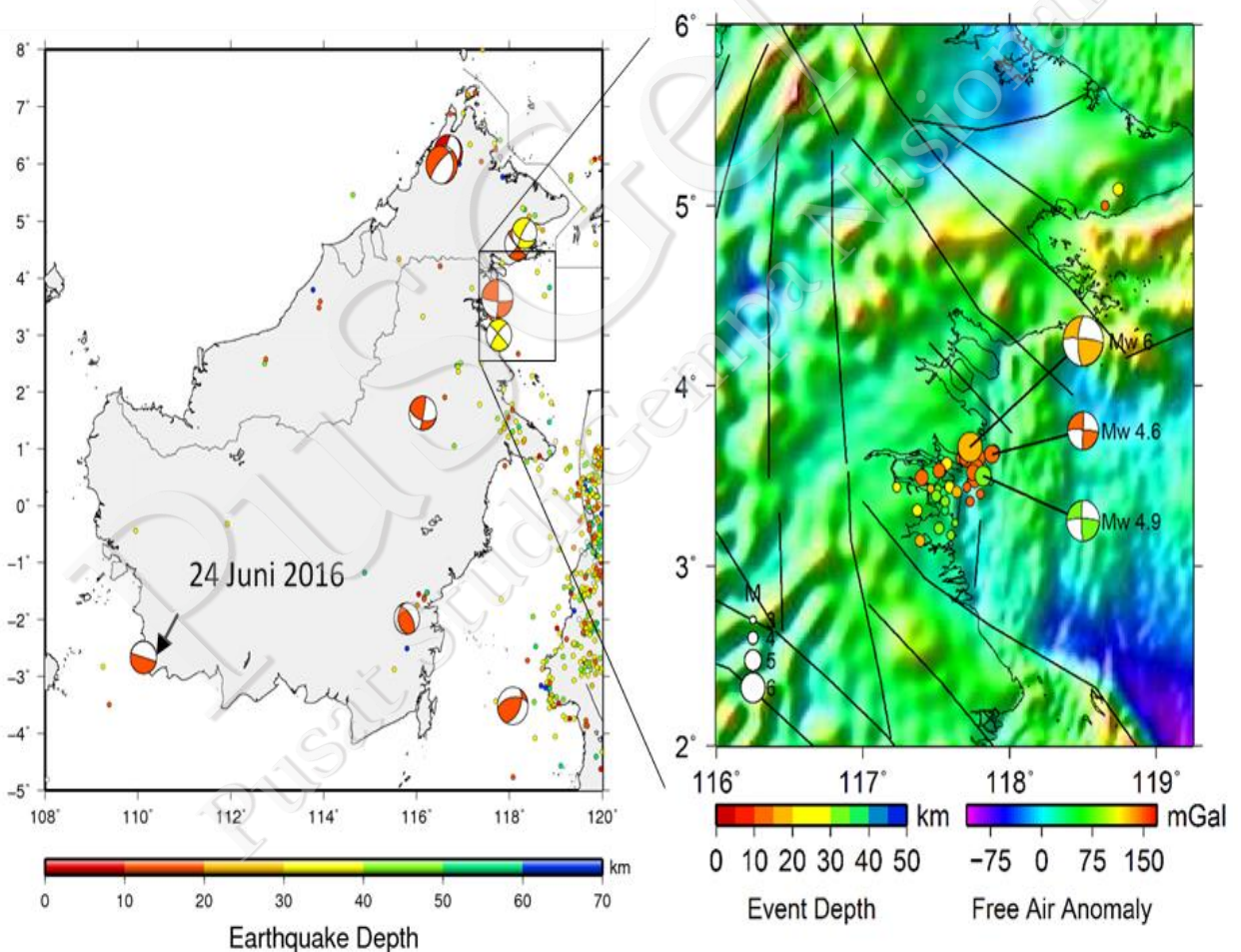
Gambar III-32. Kiri: Distribusi episenter gempa katalog PuSGeN 2017 di Pulau Kalimantan dan sekitarnya dengan magnitudo \geq 4,5 . Mekanisme fokus merupakan solusi dari GCMT untuk gempa dengan magnitudo \geq 5 dan solusi dari BMKG untuk gempa 24 Juni 2016. Sebagian besar gempa di Kalimantan diakibatkan oleh crustal fault . Kanan: Perbesaran dari wilayah Tarakan (kotak hitam) untuk mainshock dan aftershock
