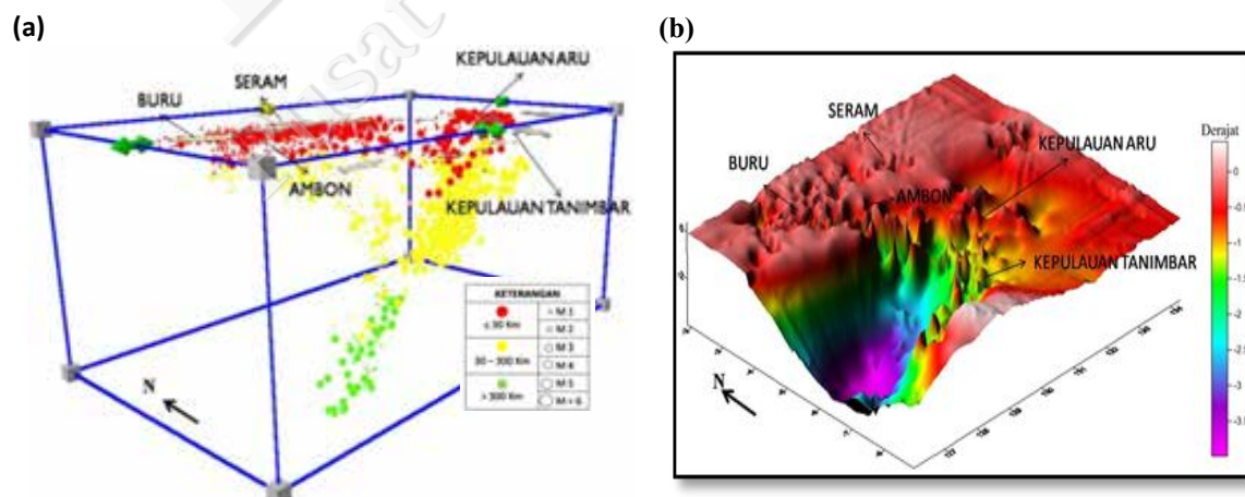
Gambar III-31. a) Peta seismisitas Laut Banda 3D. b) Interpretasi geometri slab di Laut Banda berdasarkan hiposenter gempa hasil relokasi hypoDD (Utama dkk., 2015)
