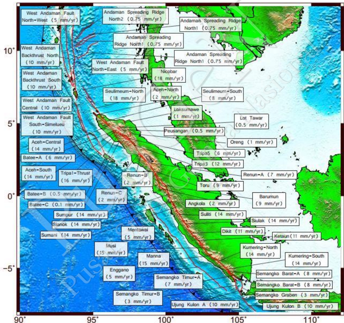
Gambar IV-27. Laju geser segmen-segmen sesar di Sumatera
