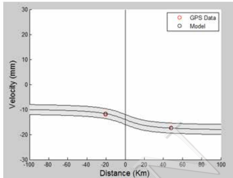
Gambar IV-21. Segmen Toru-Angkola-Barumun
