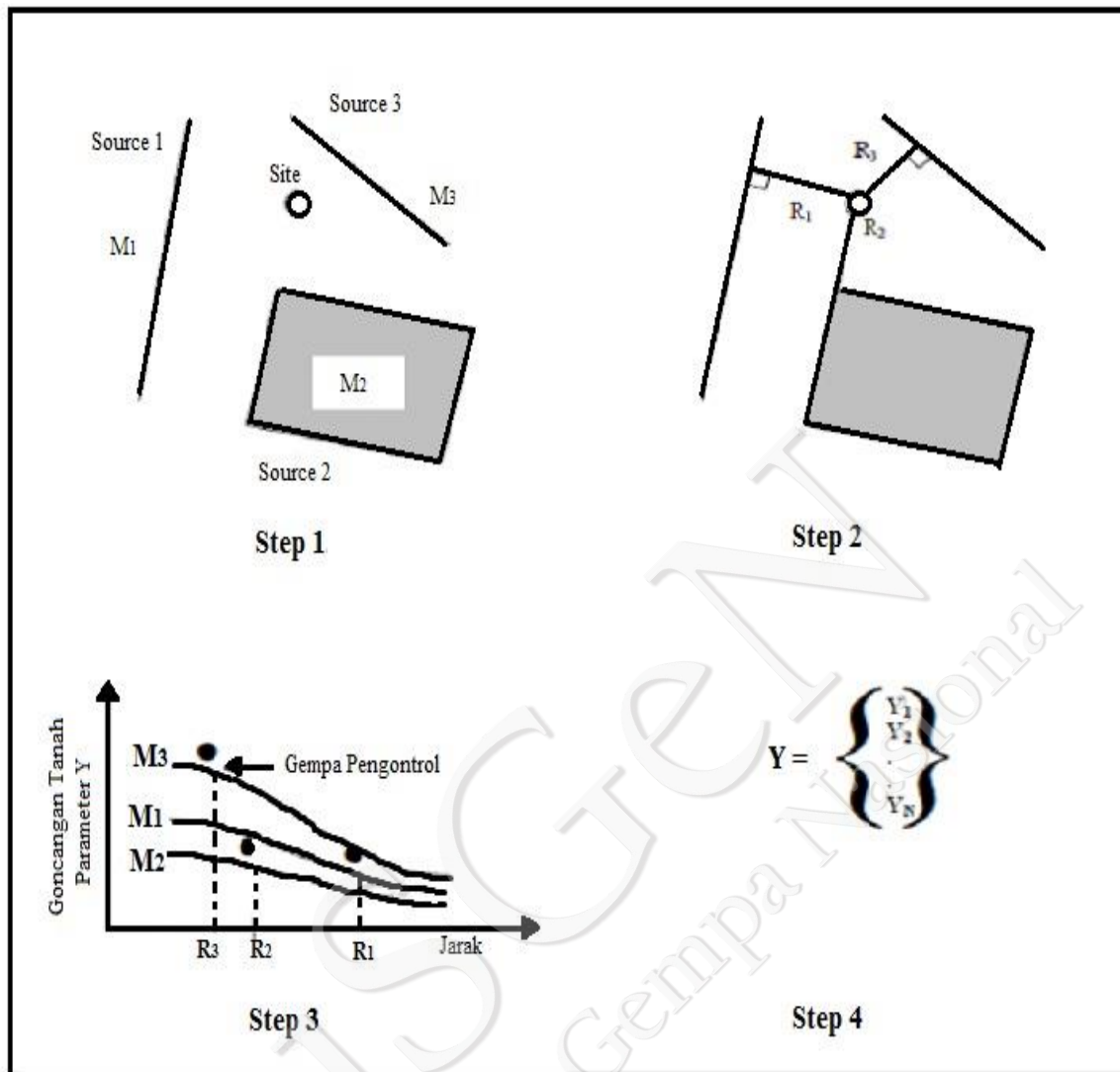
Gambar VI-2. Tahapan proses bahaya gempa dengan metode DSHA (digambar ulang dari Kramer, 1996)
