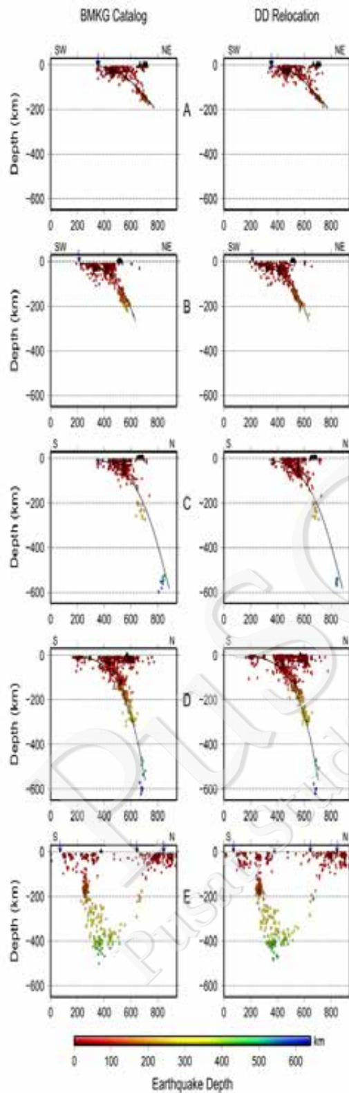
Gambar III-5. a) dan b) adalah Penampang dari hiposenter gempa hasil relokasi (simbol +) dengan magnitudo \geq 3 untuk beberapa wilayah di Indonesia. Posisi penampang ditunjukkan pada Gambar II. Segitiga hitam adalah symbol untuk gunung api dan garis hitam adalah geometri slab subduksi dari model slab 1.0 (Hayes dkk., 2012). Tanda panah berwarna biru tua adalah posisi trench
