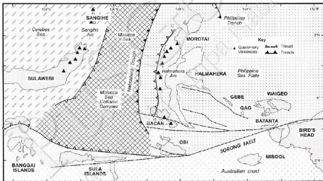
Gambar IV-47. Tektonik setting di Laut Maluku dan sekitarnya (Hall and Wilson, 2000)
