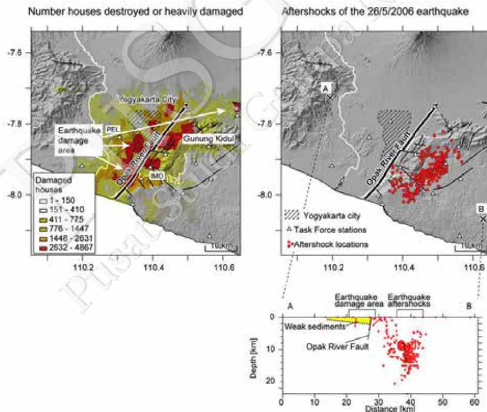
Gambar II-16. Gambar sebaran gempa susulan dari gempa Yogyakarta 2006 yang memperlihatkan sebaran membentuk bidang sesar yang berada di sebelah timur gawir Sesar Opak dan miring kearah timur (Walter dkk., 2008)
