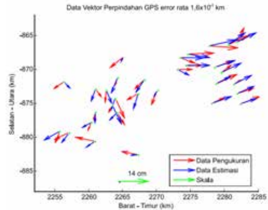
Gambar IV-77. Perhitungan laju geser Sesar Opak yang dihitung berdasarkan regangan saat gempa. Gambar sebelah kanan merupakan gambar distribusi regangan di sekitar Sesar Opak. Gambar sebelah kiri merupakan perbandingan antara vektor kecepatan titik GPS yang didapatkan dari observasi (merah) dan model (biru)
