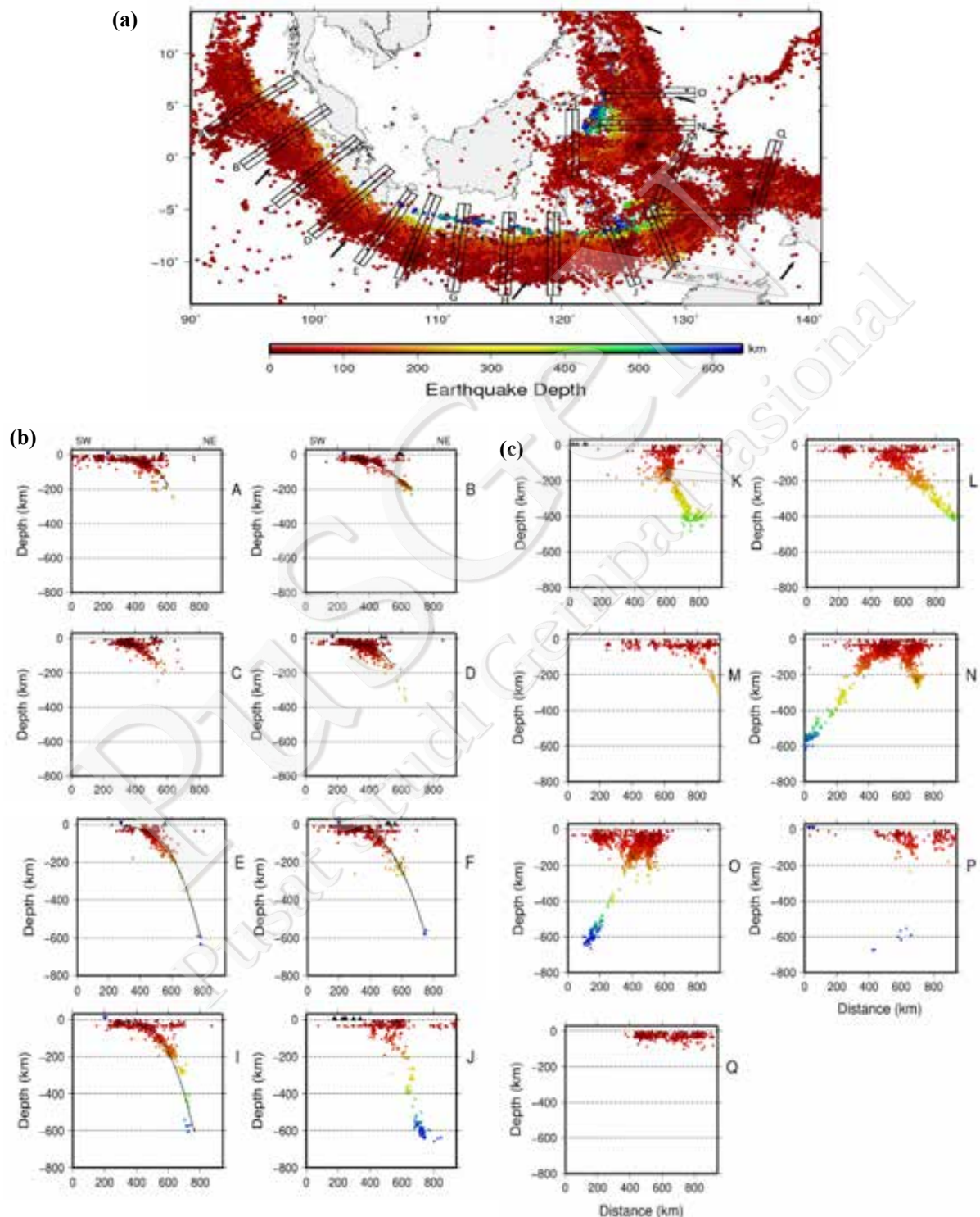
Gambar III-11. a) Penampang melintang ( cross-section ) gempa untuk beberapa zona di Indonesia. b,c) Segitiga hitam adalah simbol gunung api dan garis hitam menggambarkan geometri slab subduksi dari model slab 1.0 (Hayes dkk., 2012)
