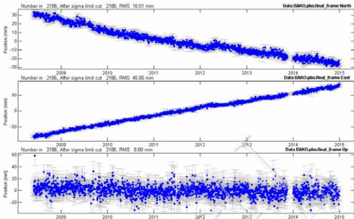
Gambar IV-11. Time series GPS di stasiun BAKO di Jawa Barat
