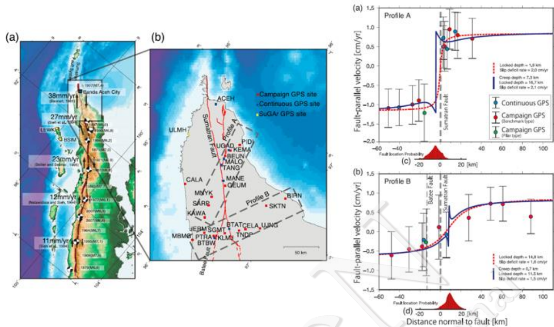
Gambar IV-19. Segmen Seulimeum-Aceh-Tripa (Ito dkk., 2012)
