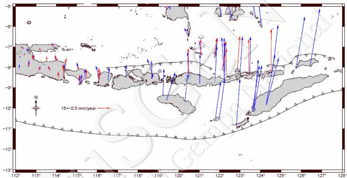
Gambar IV-54. Distribusi titik GPS dari Jawa hingga Nusa Tenggara yang terdiri atas GPS berkala dan GPS kontinyu (Susilo dkk. 2016)
