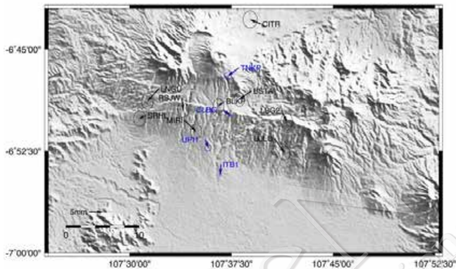
Gambar IV-31. Vektor pergerakan titik GPS yang digunakan dalam perhitungan laju geser Sesar Lembang (Meilano dkk, 2012)
