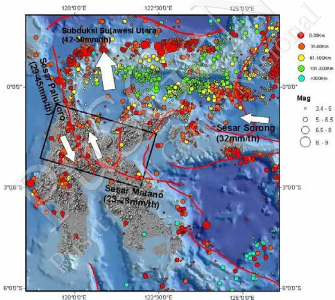
Gambar II-18. Struktur Geologi Regional di Pulau Sulawesi (Daryono, 2016). Vektor pergerakan adalah kompilasi hasil penelitian geodesi deformasi di Sulawesi. Peta dasar menggunakan SRTM 90 m dan ETOPO1
