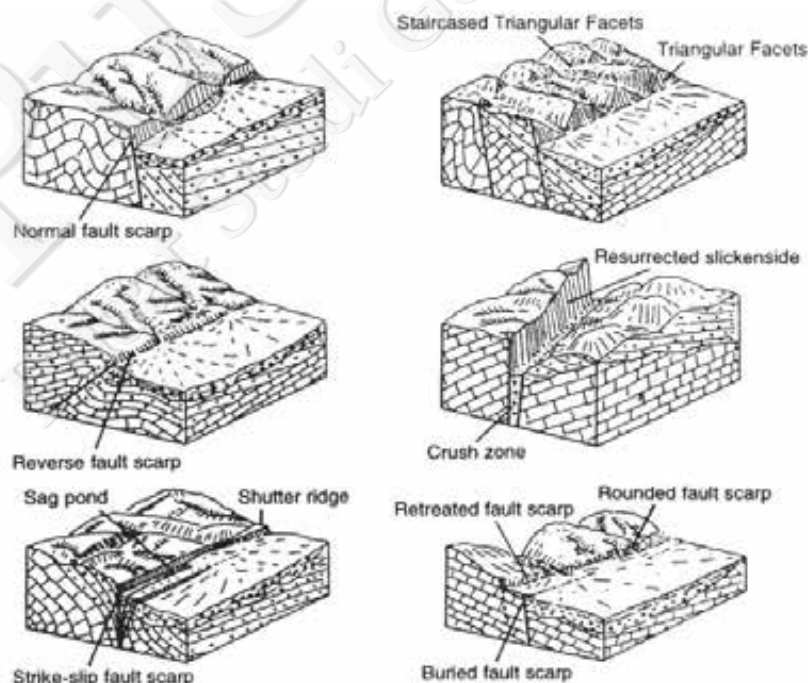
Gambar II-1. Bentuk morfologi yang berhubungan dengan sesar aktif. Bentuk-bentuk tersebut diberi simbol berdasarkan morfologi yang muncul (McCalpin, 1996)
