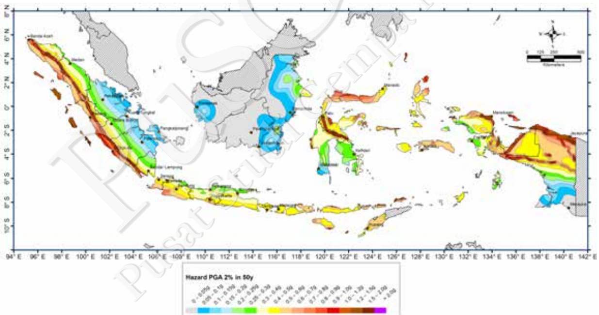
Gambar VI-20. Peta percepatan puncak di batuan dasar (SB) untuk probabilitas terlampaui 2% dalam 50 tahun
