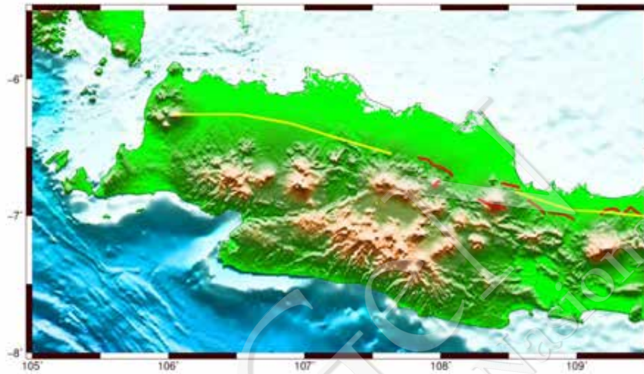
Gambar IV-33. Sesar Baribis yang terletak di wilayah Jawa Barat. Garis dengan warna merah mengindikasikan segmen Sesar Baribis yang diajukan oleh Pokja Geologi. Garis berwarna kuning merupakan garis Sesar Baribis yang diajukan oleh Koulali dkk, 2016
