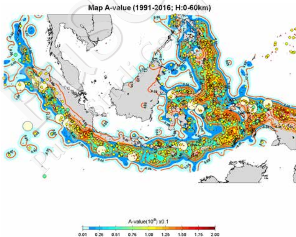
Gambar III-7. (a) Peta a-value untuk data gempa dengan kedalaman fokus kurang dari atau sama dengan 60 km dari tahun 1963-1990. (b) Peta a-value untuk data gempa dari tahun 1991-2016. Hasil a-value dari kedua periode tersebut memberikan pola yang cukup mirip
