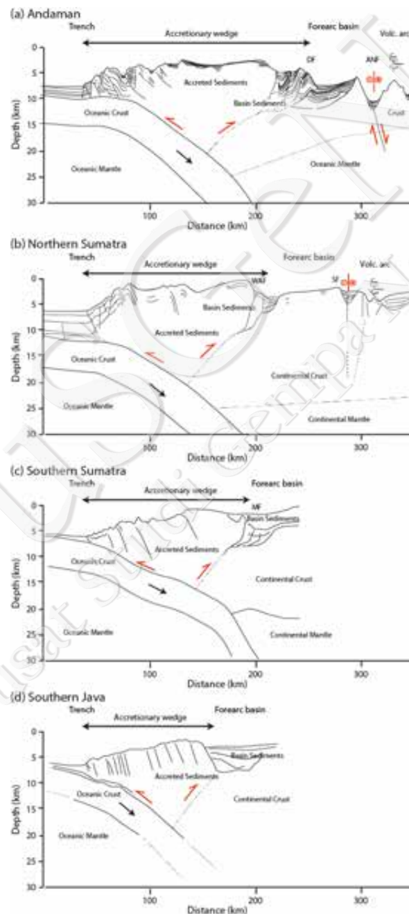
Gambar II-10. Kompleks prisma akresi di sepanjang tepian barat Sundaland. Dimensi prisma akresi makin menyempit ke arah selatan Jawa (Modifikasi dari Kopp dkk., 2009; Singh dkk., 2011; Singh dkk., 2013)
