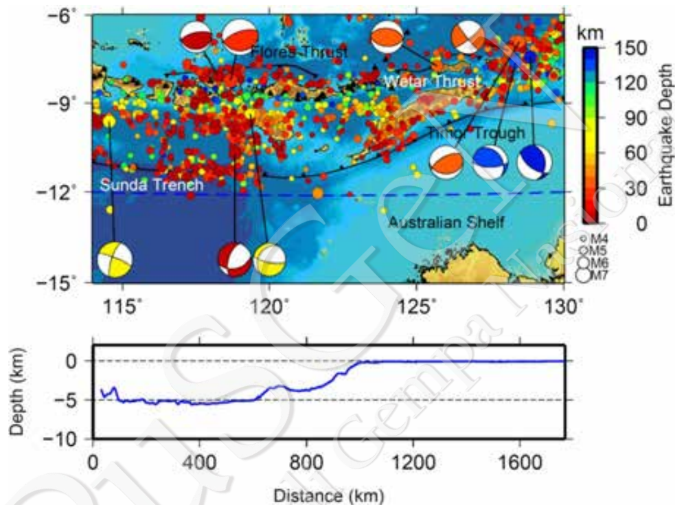
Gambar III-29. Atas: Episenter gempa hasil relokasi di zona transisi Sunda-Banda dan sekitarnya untuk event dengan kedalaman \leq 150 km dan magnitudo \geq 4 . Mekanisme fokus merupakan solusi dari GCMT untuk gempa dengan magnitudo \geq 6 . Garis biru putus-putus adalah posisi penampang data batimetri permukaan laut. Bawah: penampang vertikal dari data batimetri SRTM 15 (Shiddiqi, 2015).
