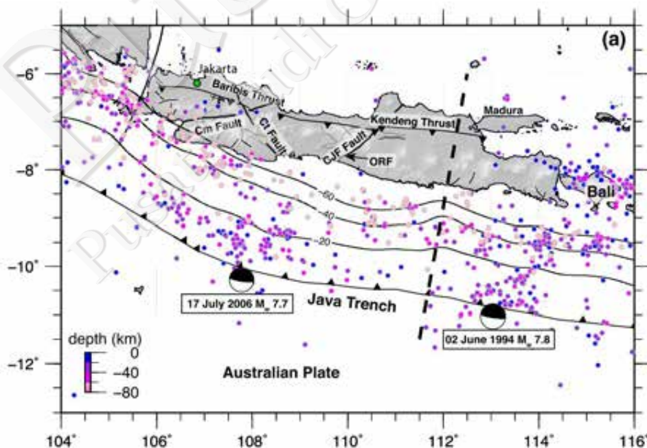
Gambar IV-38. Sesar Kendeng yang terletak memanjang sepanjang Jawa Timur dan Jawa Tengah menurut Koulali dkk (2016)
