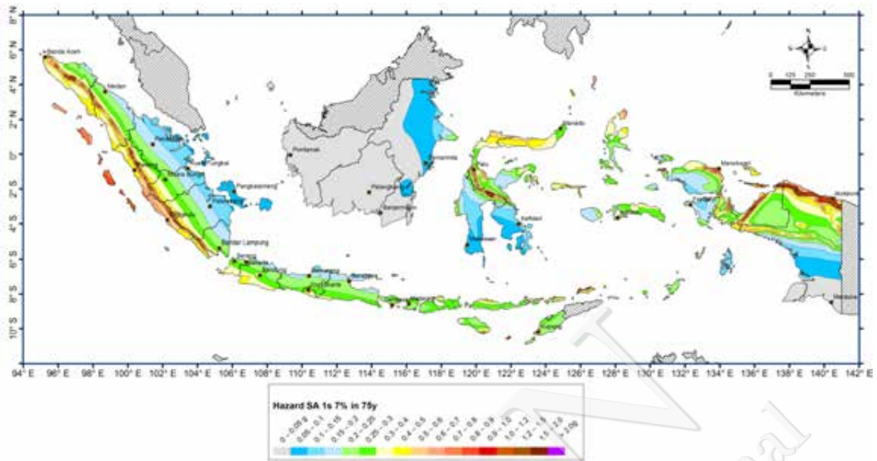
Gambar VI-19. Peta percepatan spektrum respons 1.0 detik dengan nisbah redaman 5% di batuan dasar (SB) untuk probabilitas terlampaui 7% dalam 75 tahun
